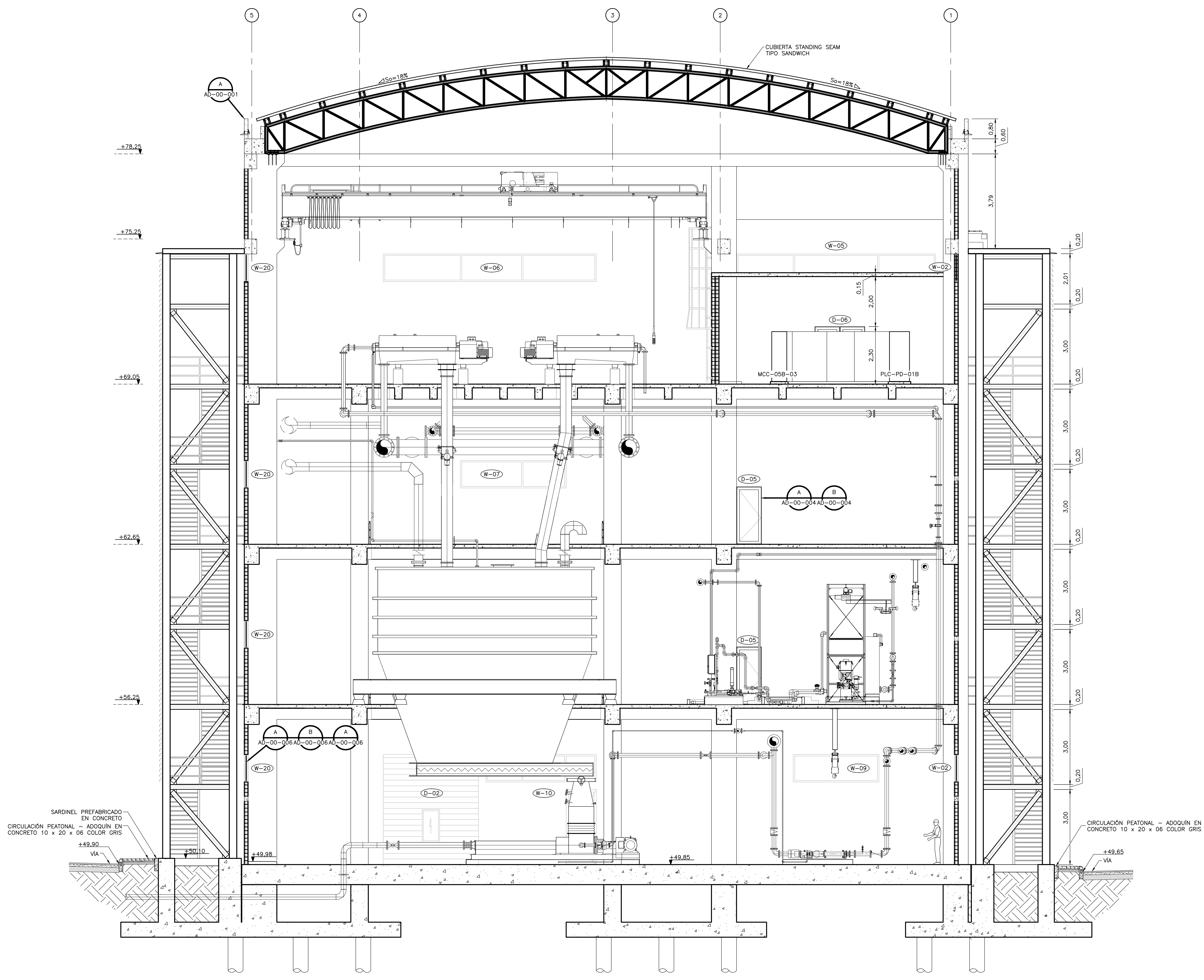
SECCIÓN 2 2 2 2 2 1=75 A-05-020 A-05-021 A-05-022 A-05-023 A-05-024
