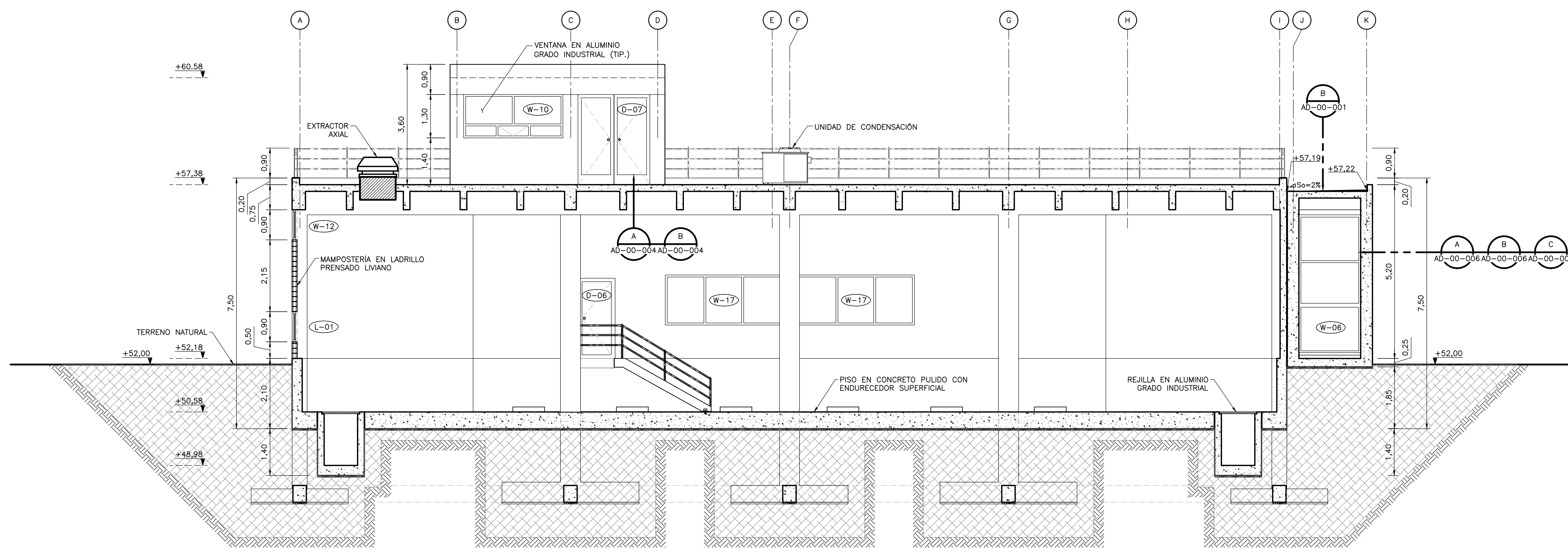
SECCIÓN 2 1=75 A-07-001 A-07-002 A-07-003
