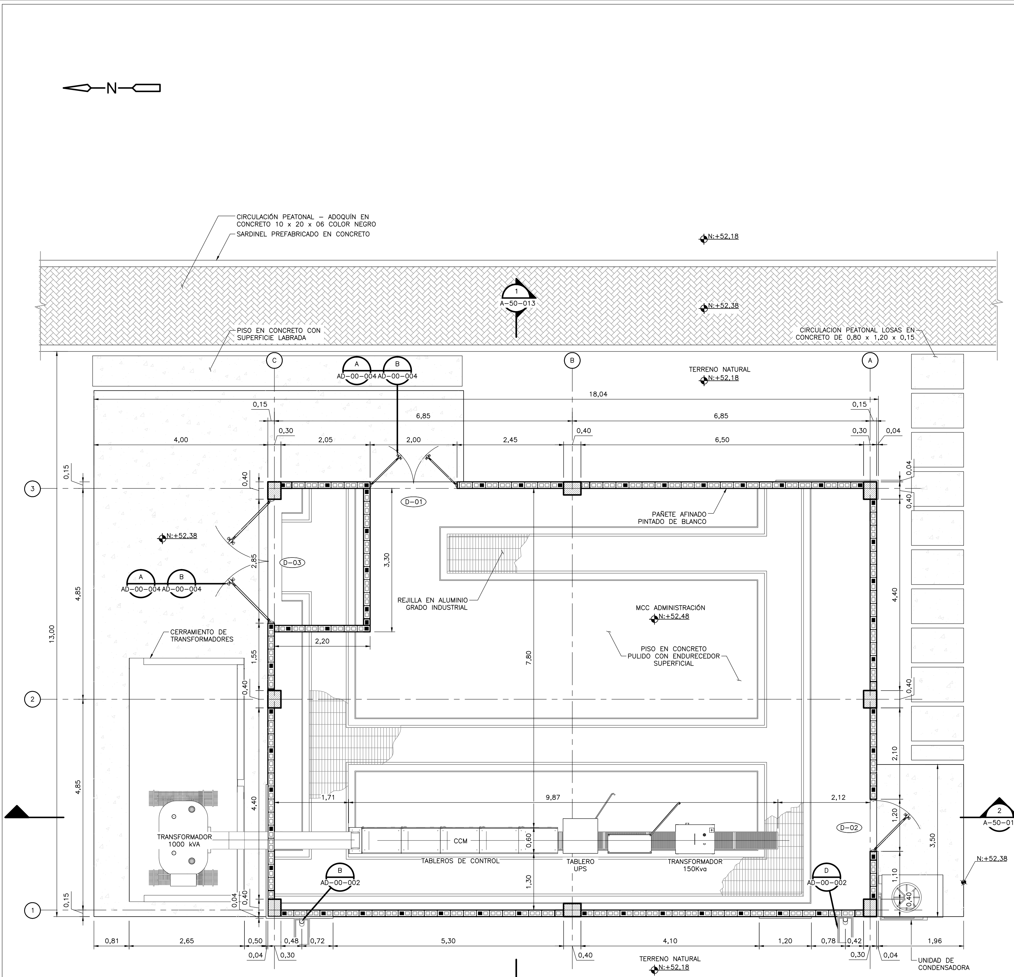
PLANTA PRIMER PISO 1=50
