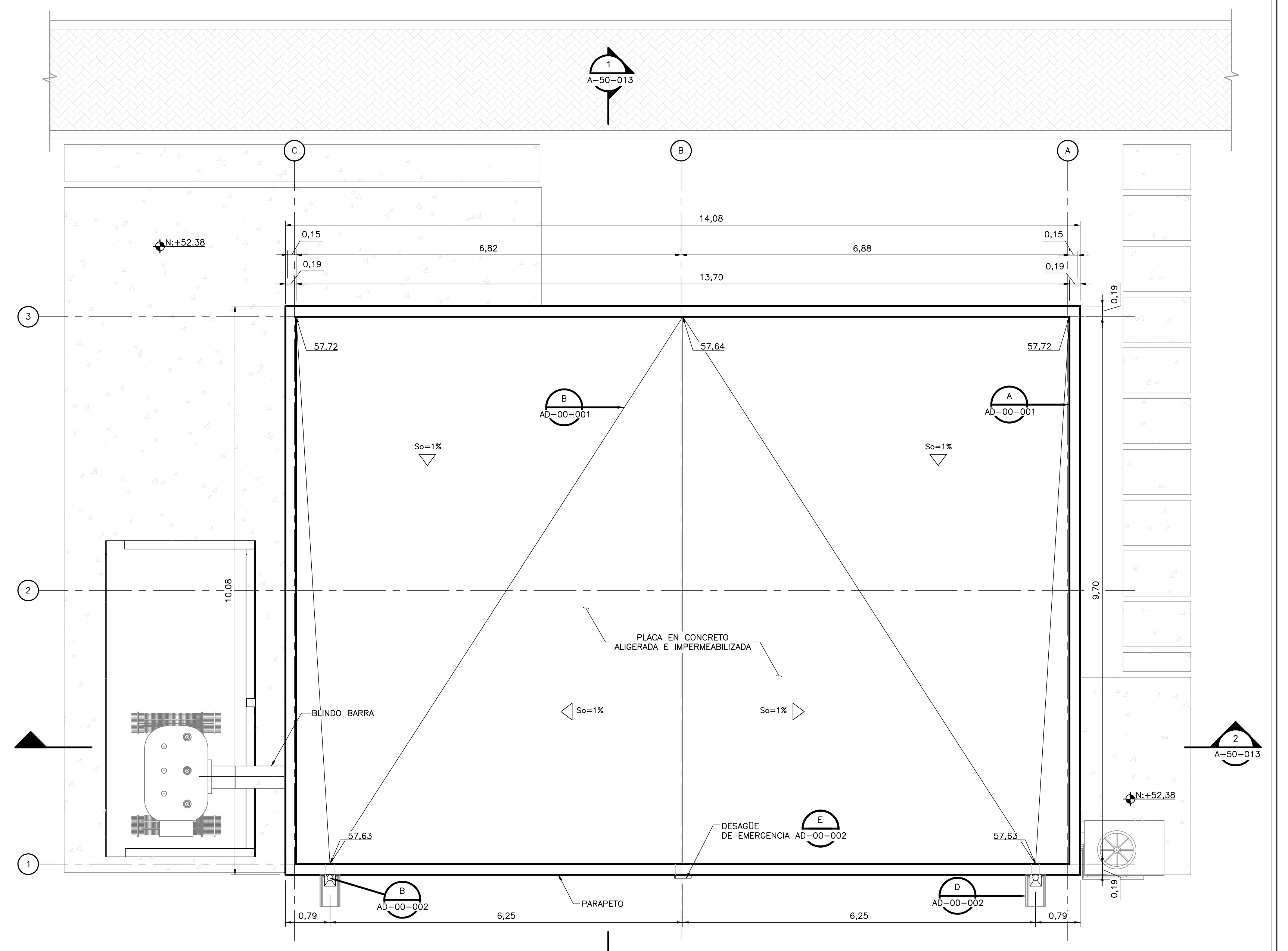
PLANTA CUBIERTA 1=50
