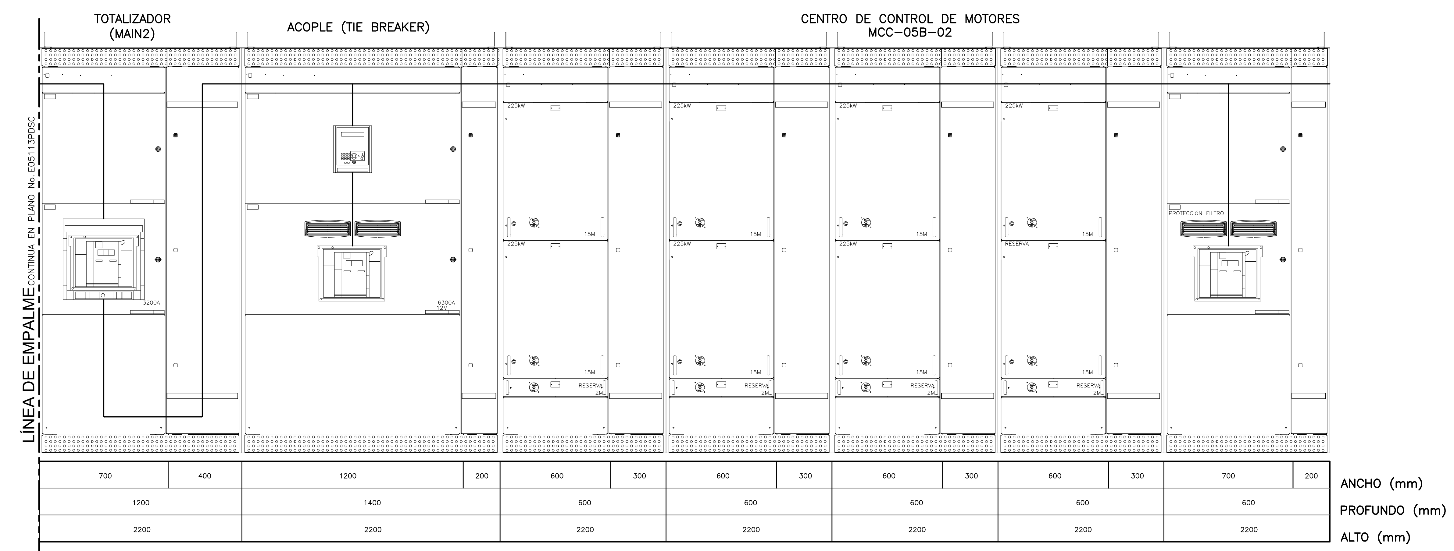
ALZADO 2 SIN ESCALA E-05-111
