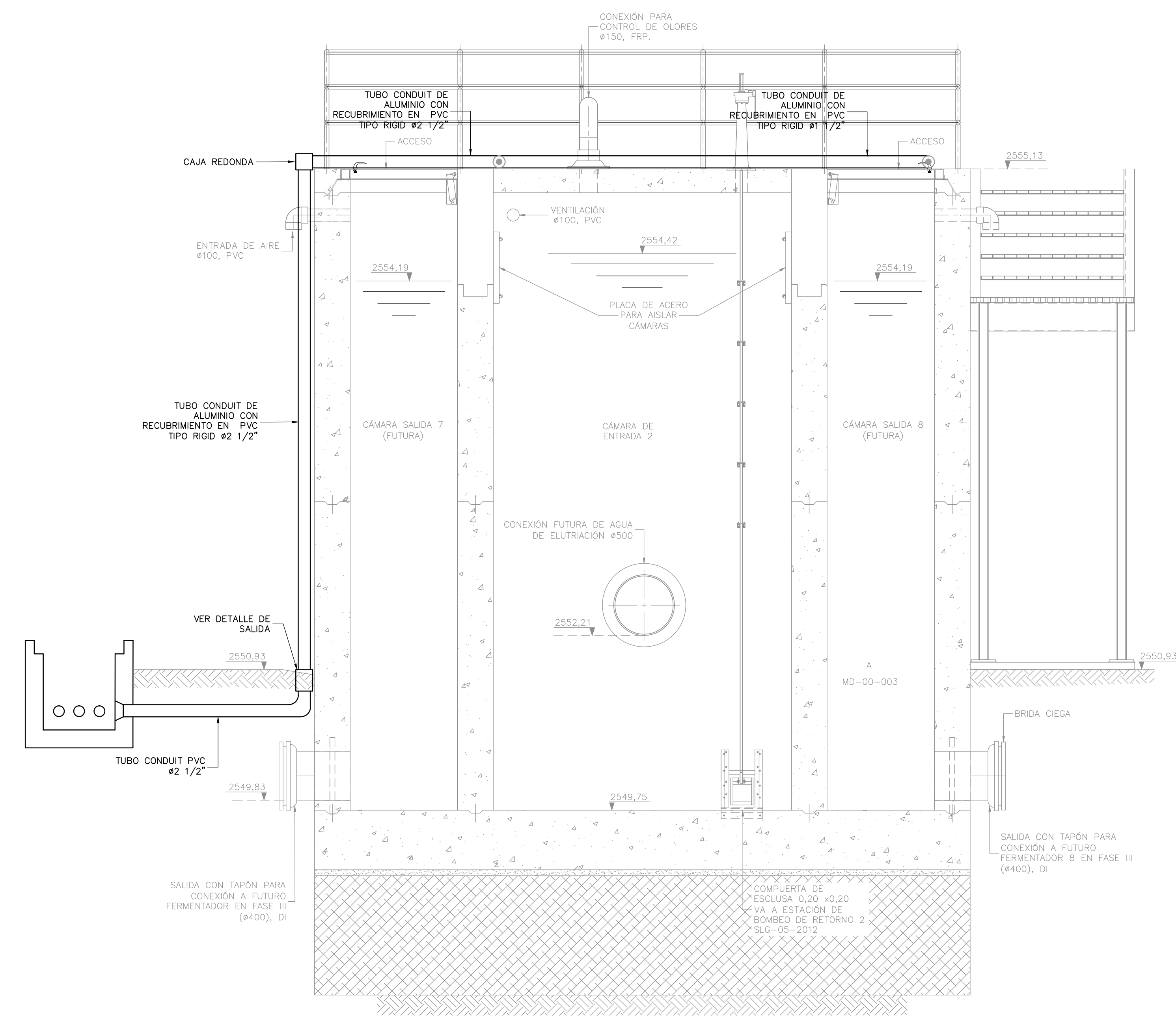
INSTALACIÓN DE TUBERÍA SECCIÓN 1 1=25 E-05-219E
