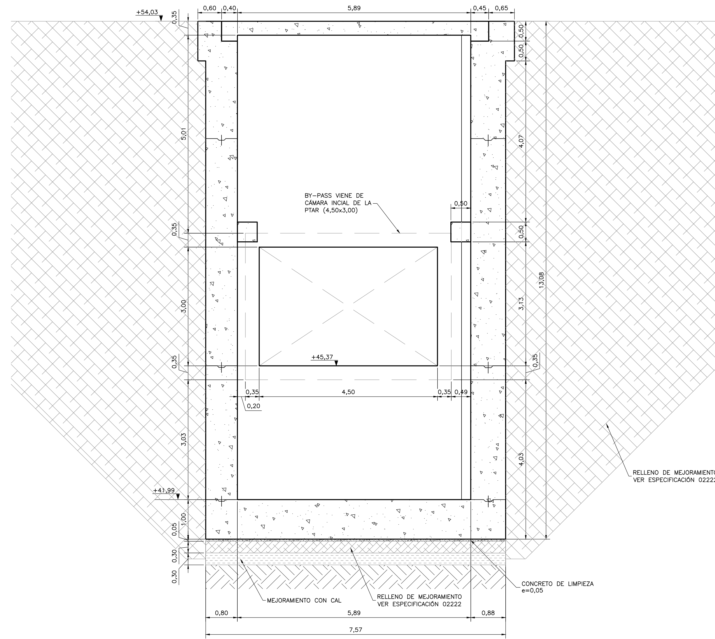
SECCIÓN 3 1=75 S-04-064
