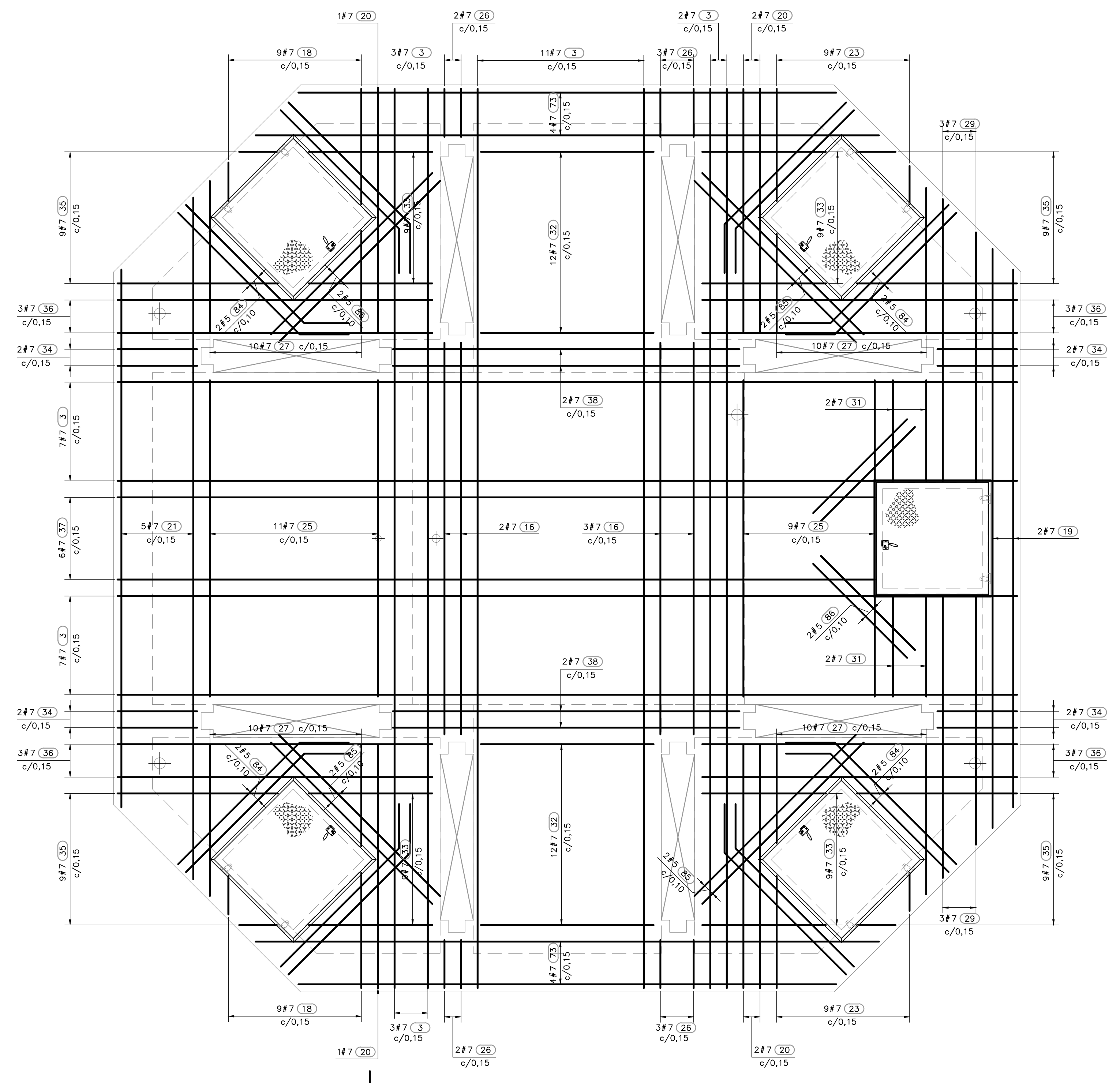
REFUERZO INFERIOR Y SUPERIOR PLANTA PLACA SUPERIOR 1=25
