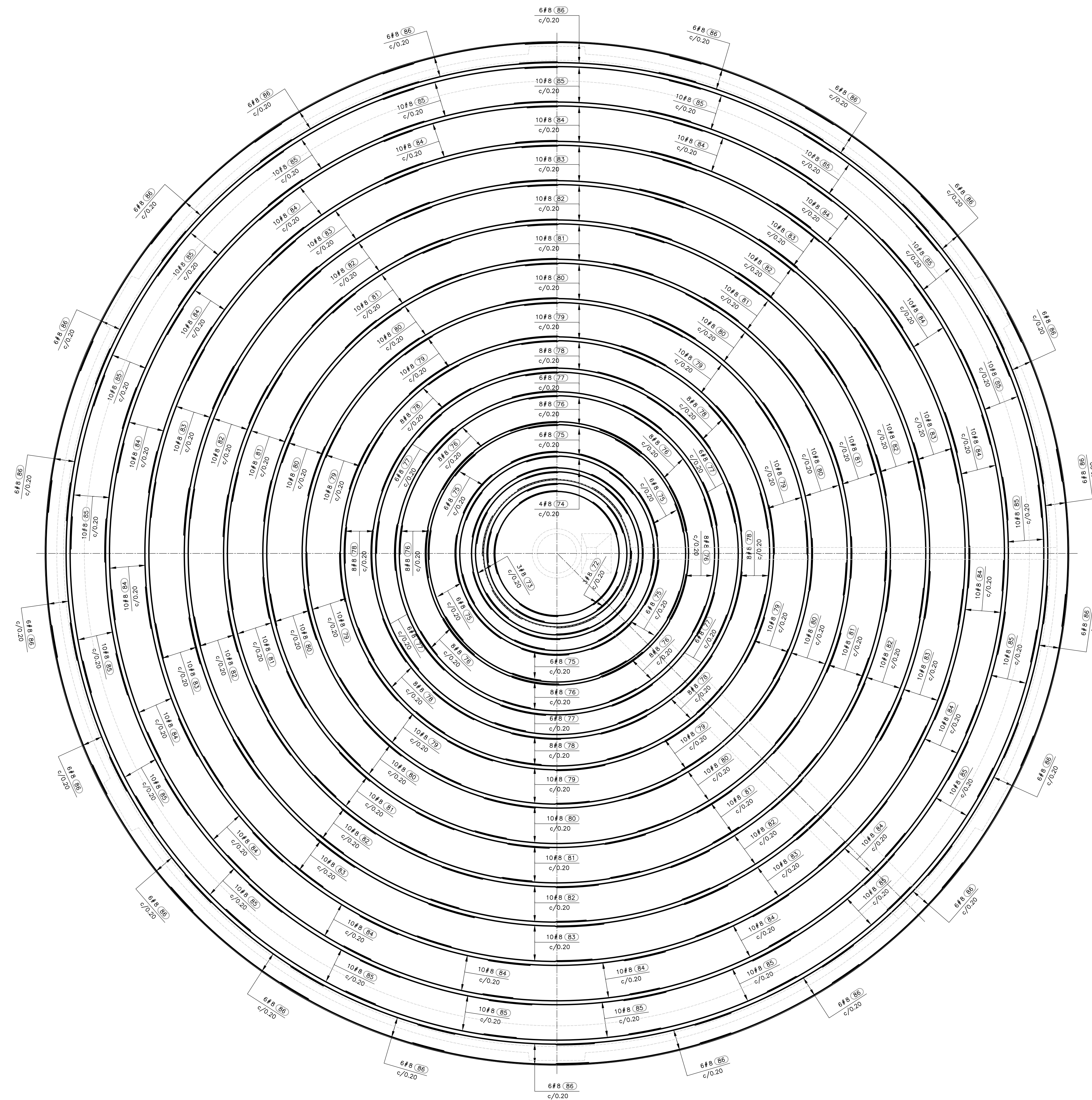
REFUERZO CIRCULAR CARA SUPERIOR E INFERIOR SEDIMENTADORES 1 Y 4 PLANTA PLACA DE FONDO 1=100
