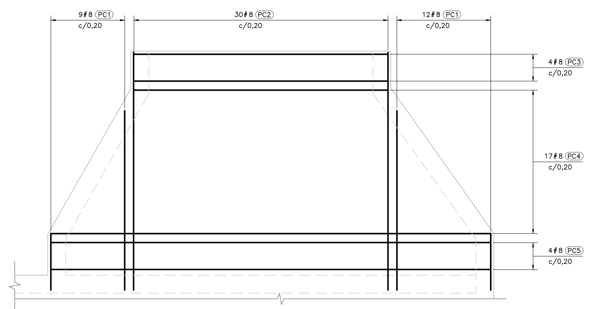
REFUERZO SUPERIOR E INFERIOR PLANTA SUPERIOR CONDUCTO DE SALIDA 1=50
