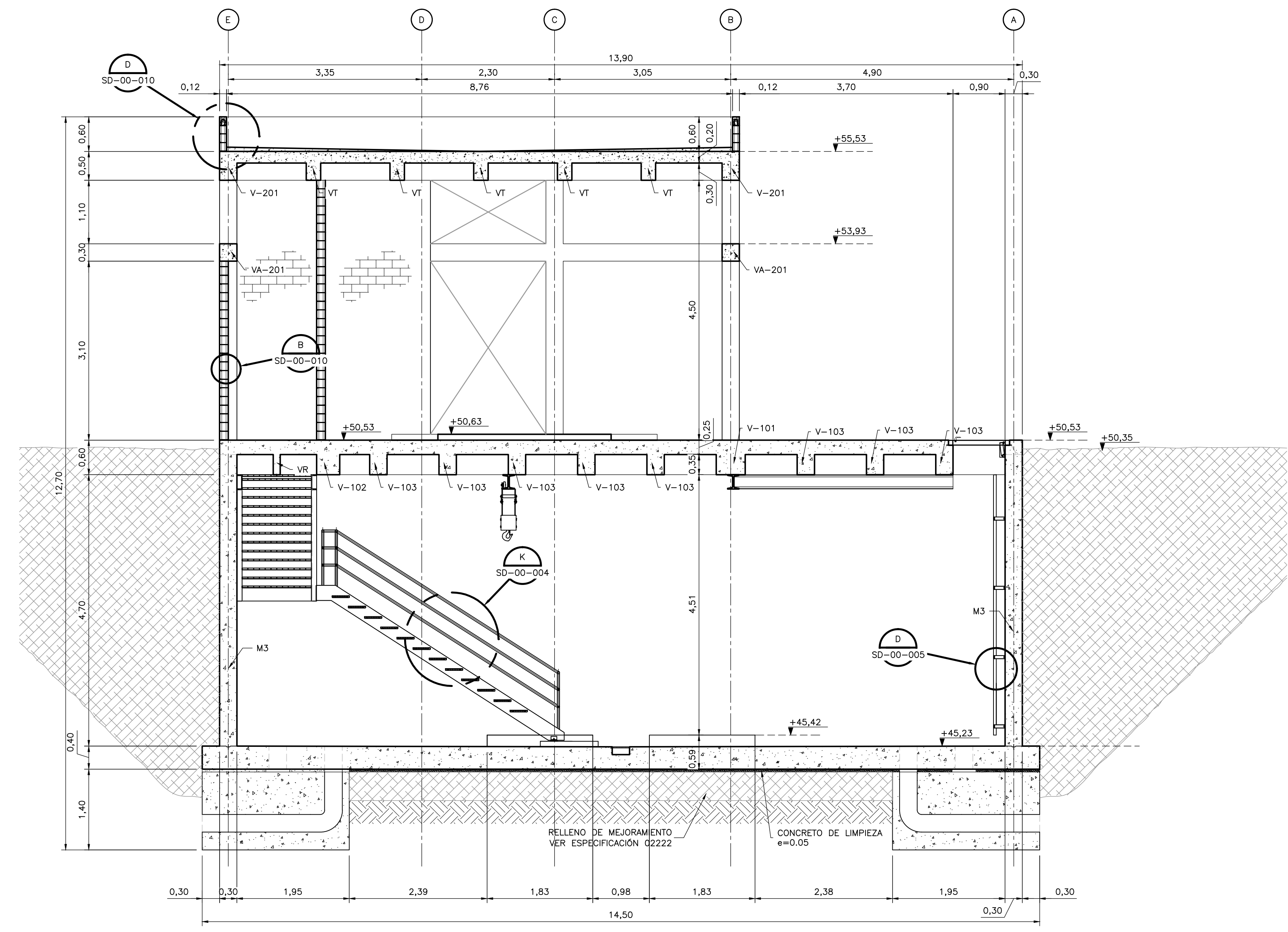
SECCIÓN 1 1 1=50 S-04-070 S-04-071
