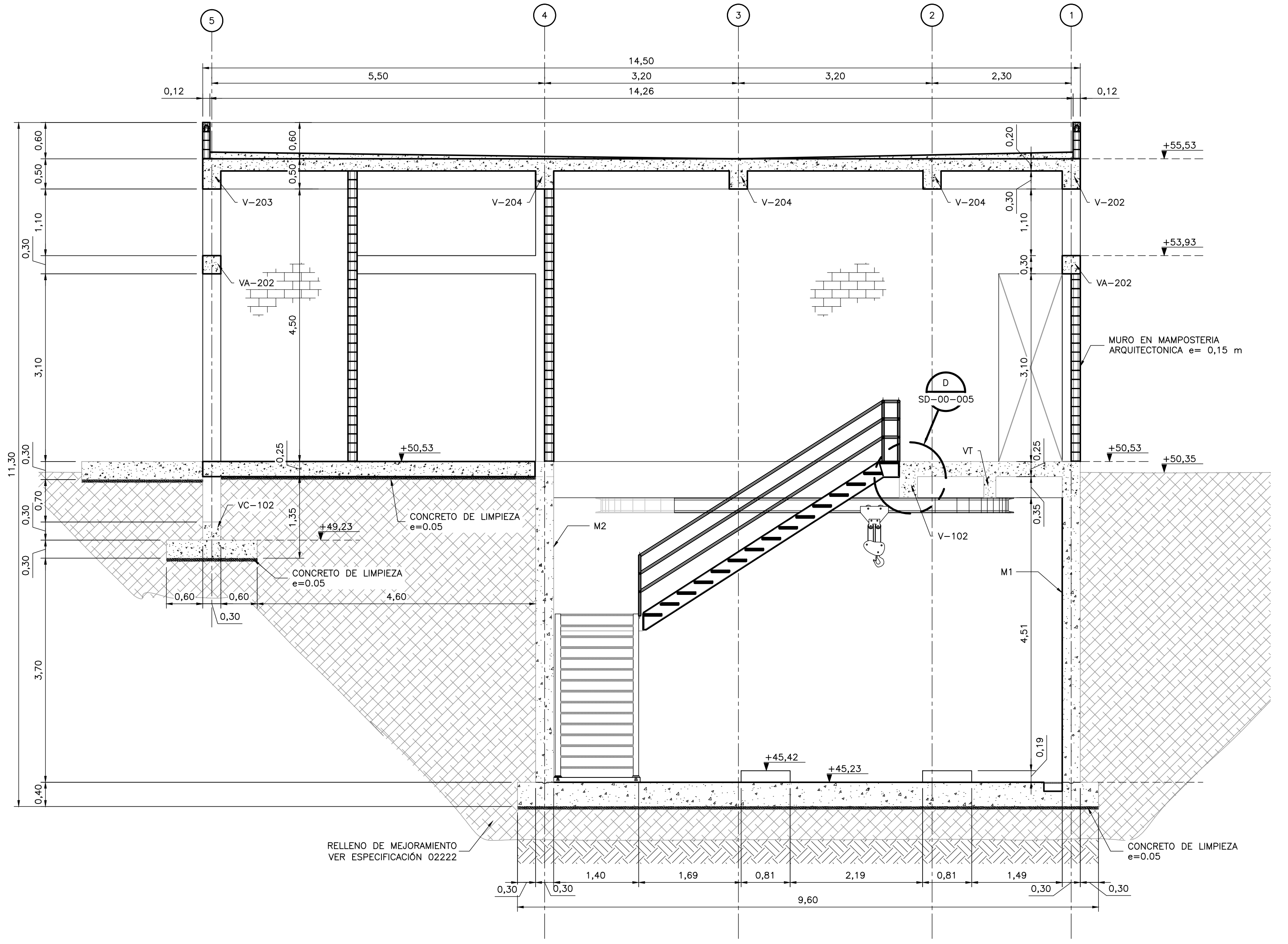
SECCIÓN 2 2 1=50 S-04-070 S-04-071
