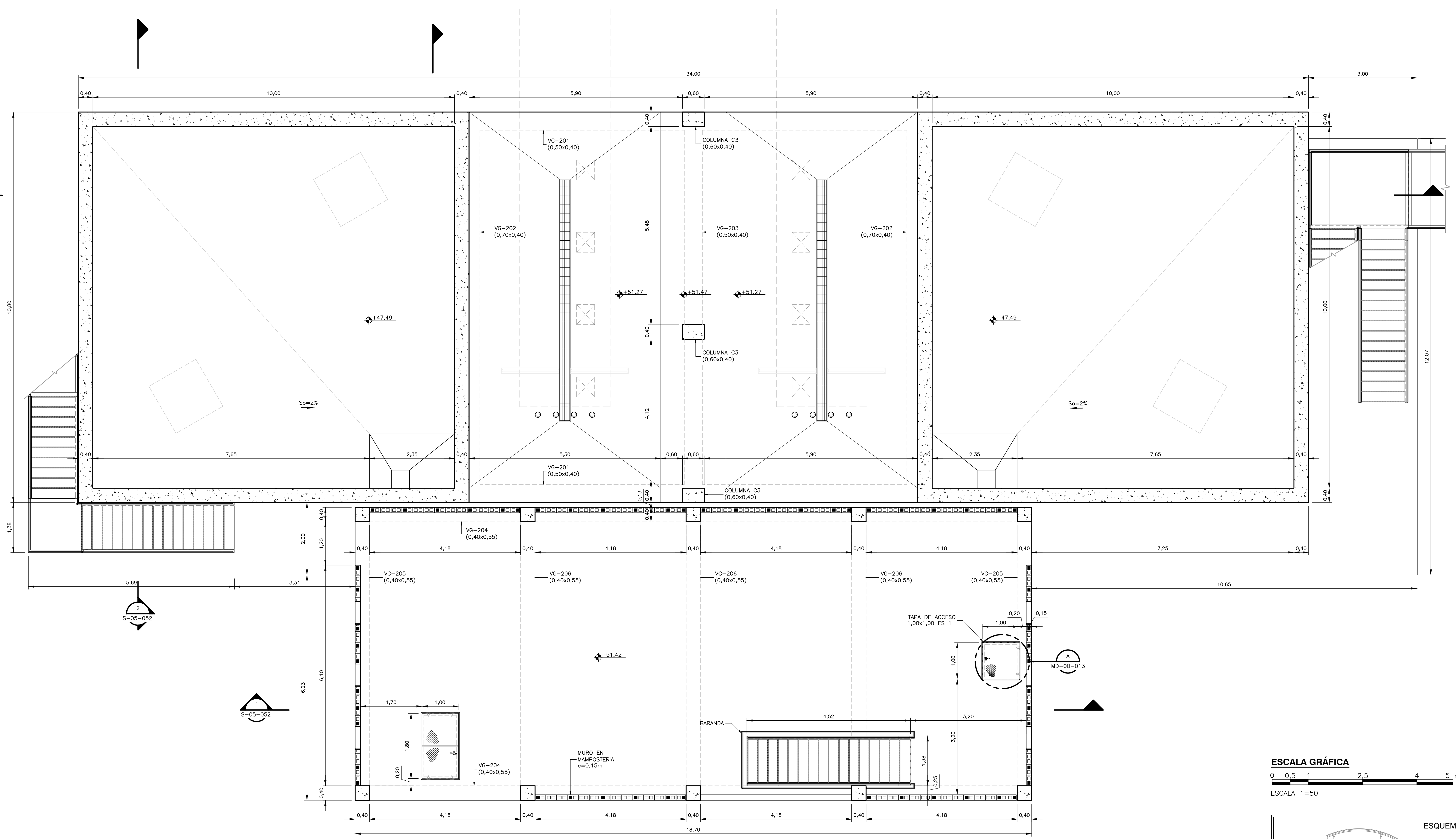
PLANTA INTERMEDIA 1=50
