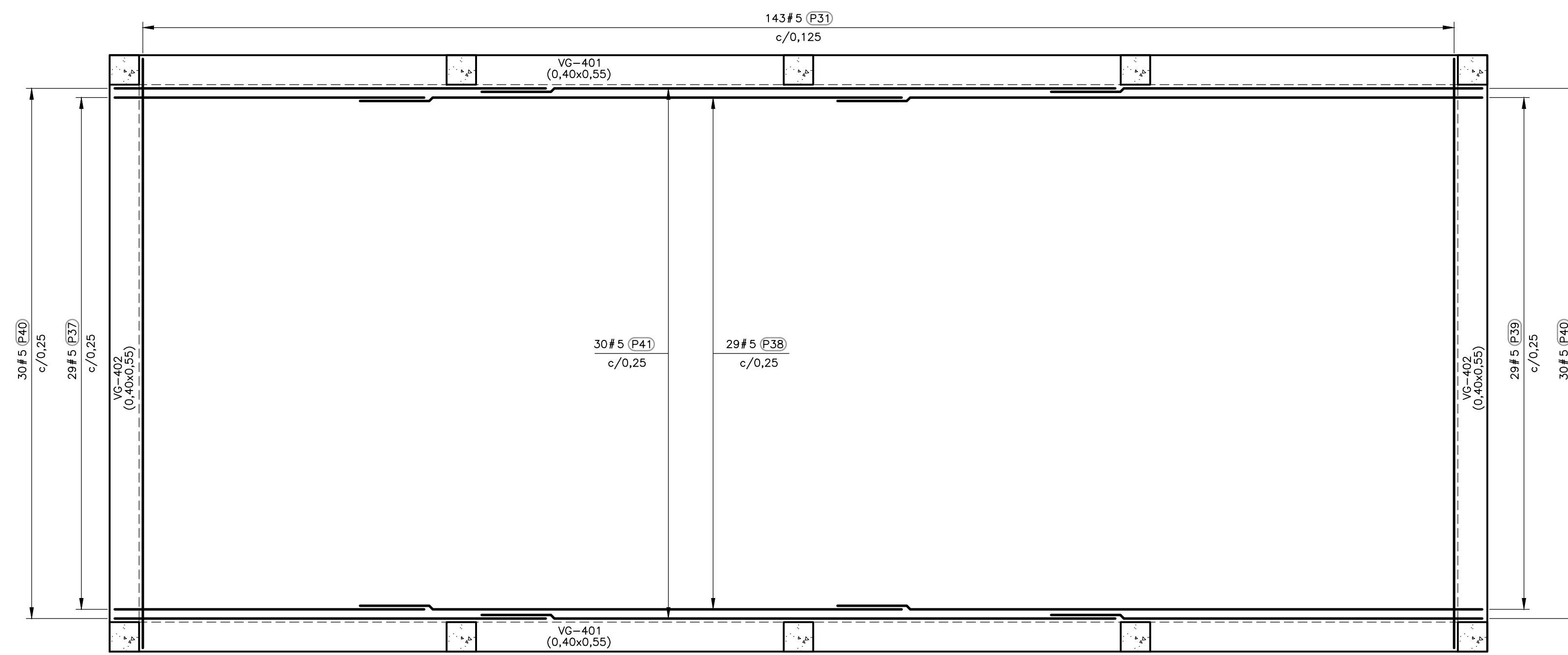
LOSA 3 CUARTO DE BOMBAS REFUERZO INFERIOR 1=50
