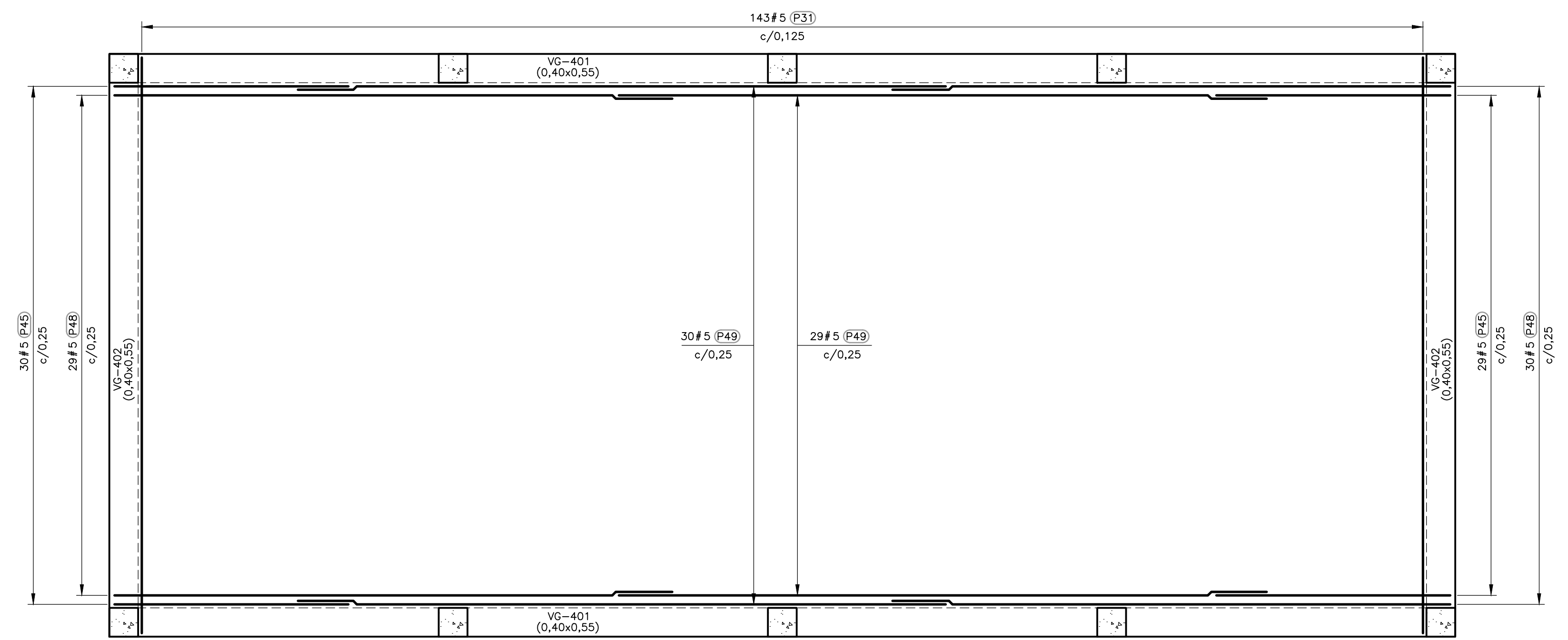
LOSA 3 CUARTO DE BOMBAS REFUERZO SUPERIOR 1=50
