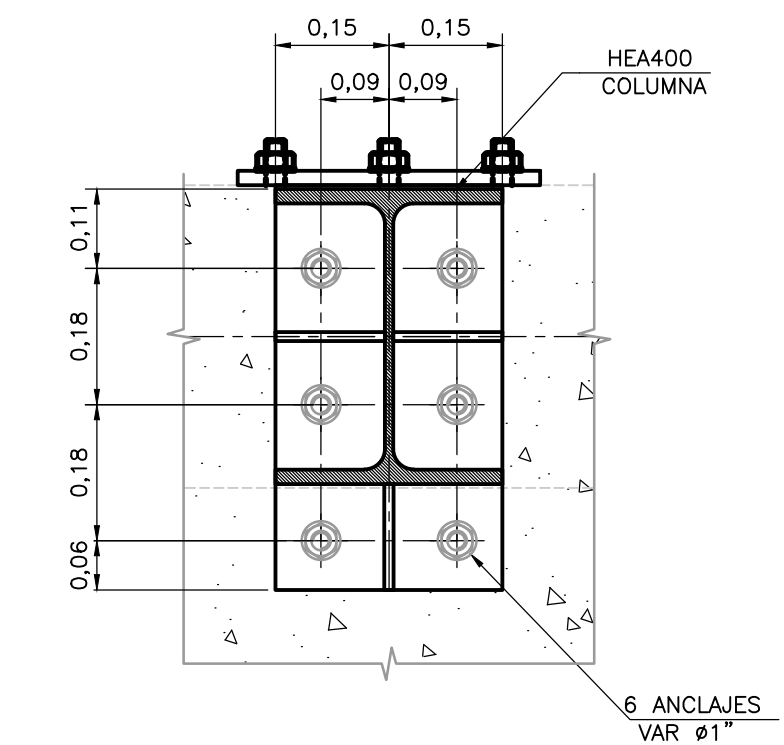
UBICACIÓN DE ANCLAJES DETALLE A 1=10 S-05-063
