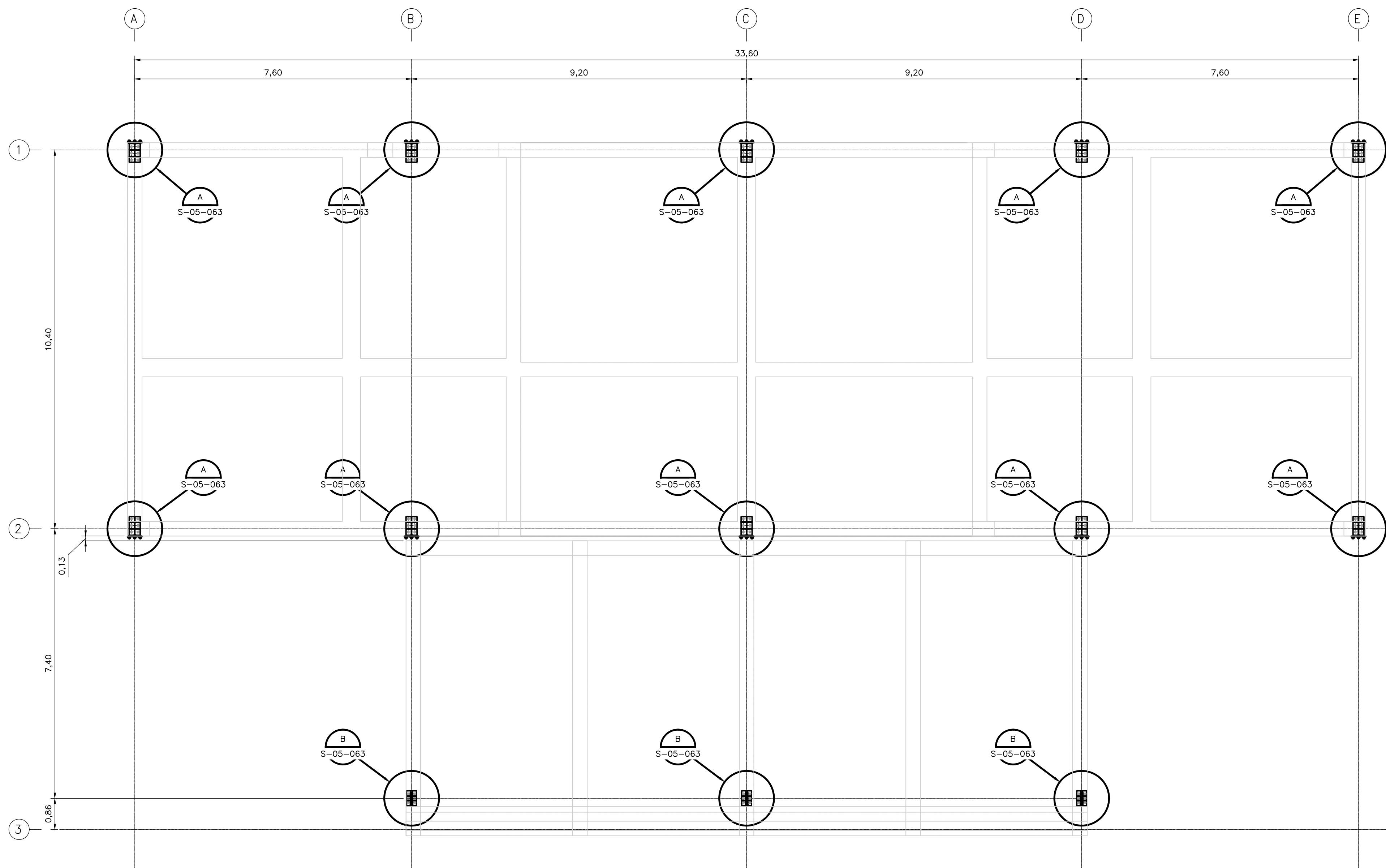
ESTRUCTURA CRIBADO LODOS Y NATAS PLANTA LOCALIZACION COLUMNAS
