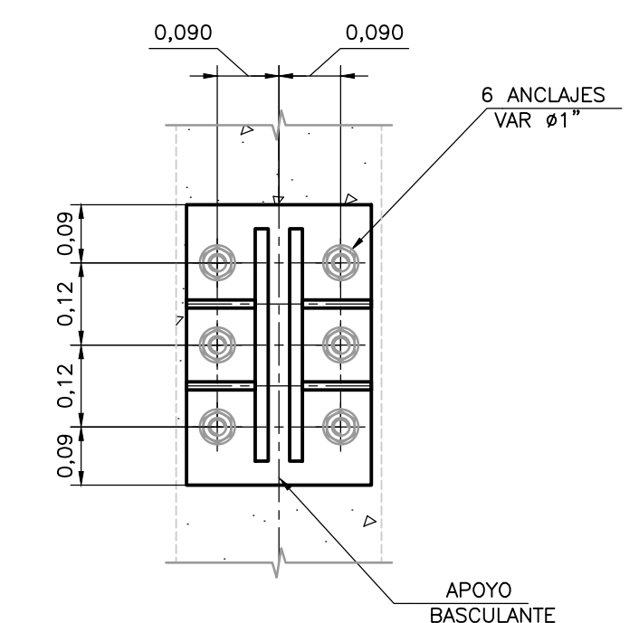
UBICACIÓN DE ANCLAJES DETALLE B 1=10 S-05-063
