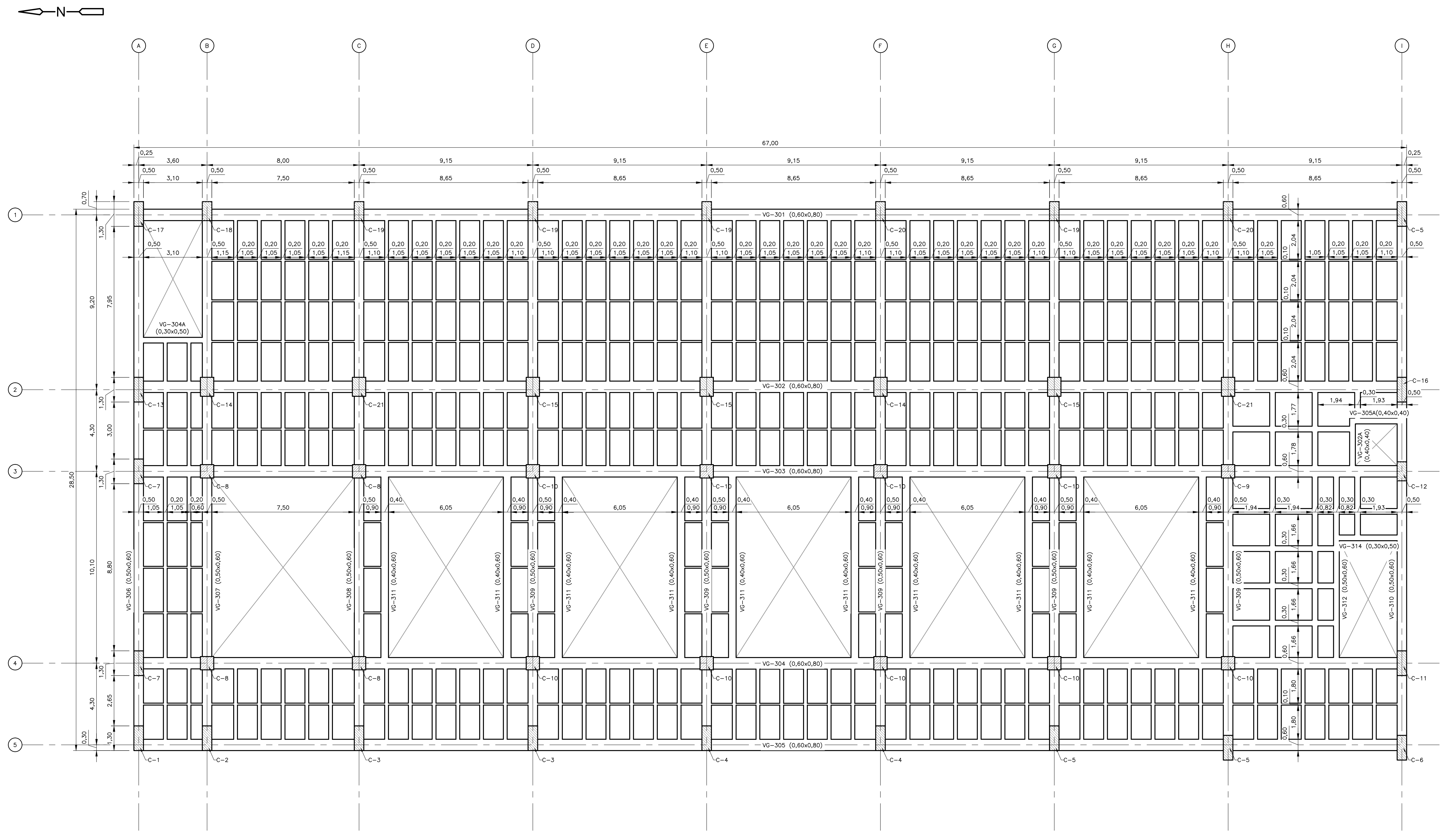
PLACA ENTREPISO TERCER PISO 1 = 100
