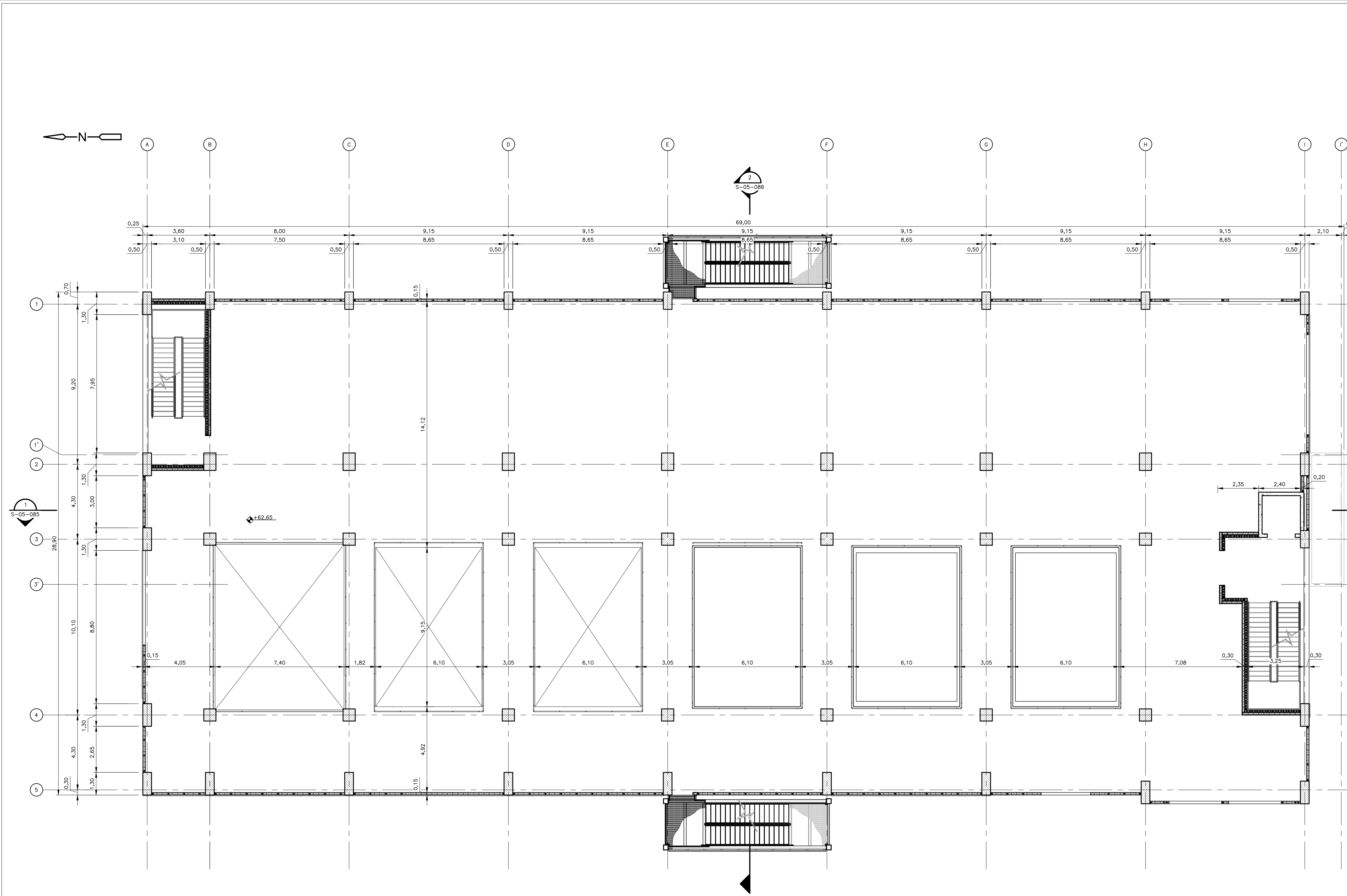
PLANTA TERCER PISO 1 = 100
