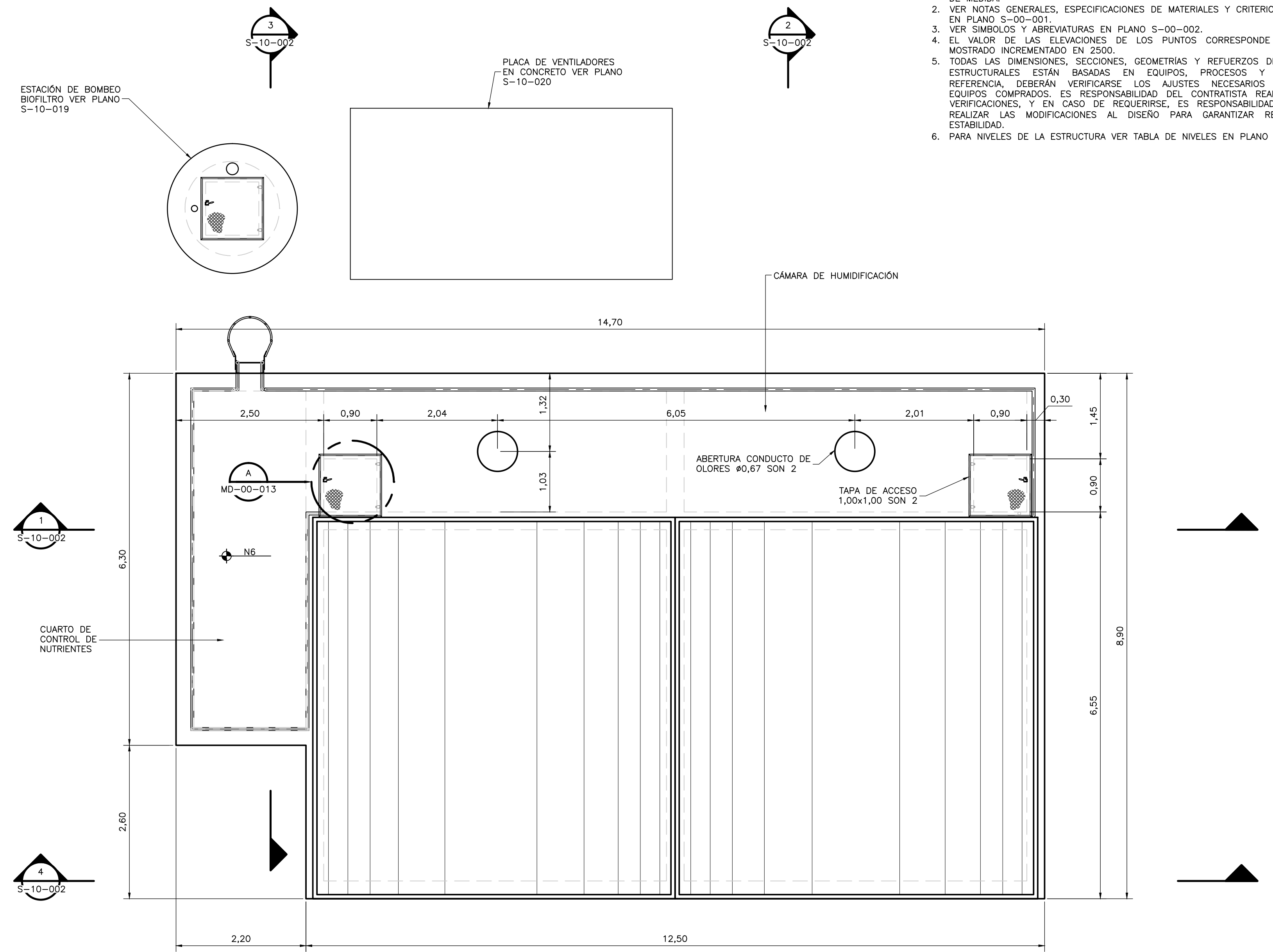
PLANTA SUPERIOR 1:50
