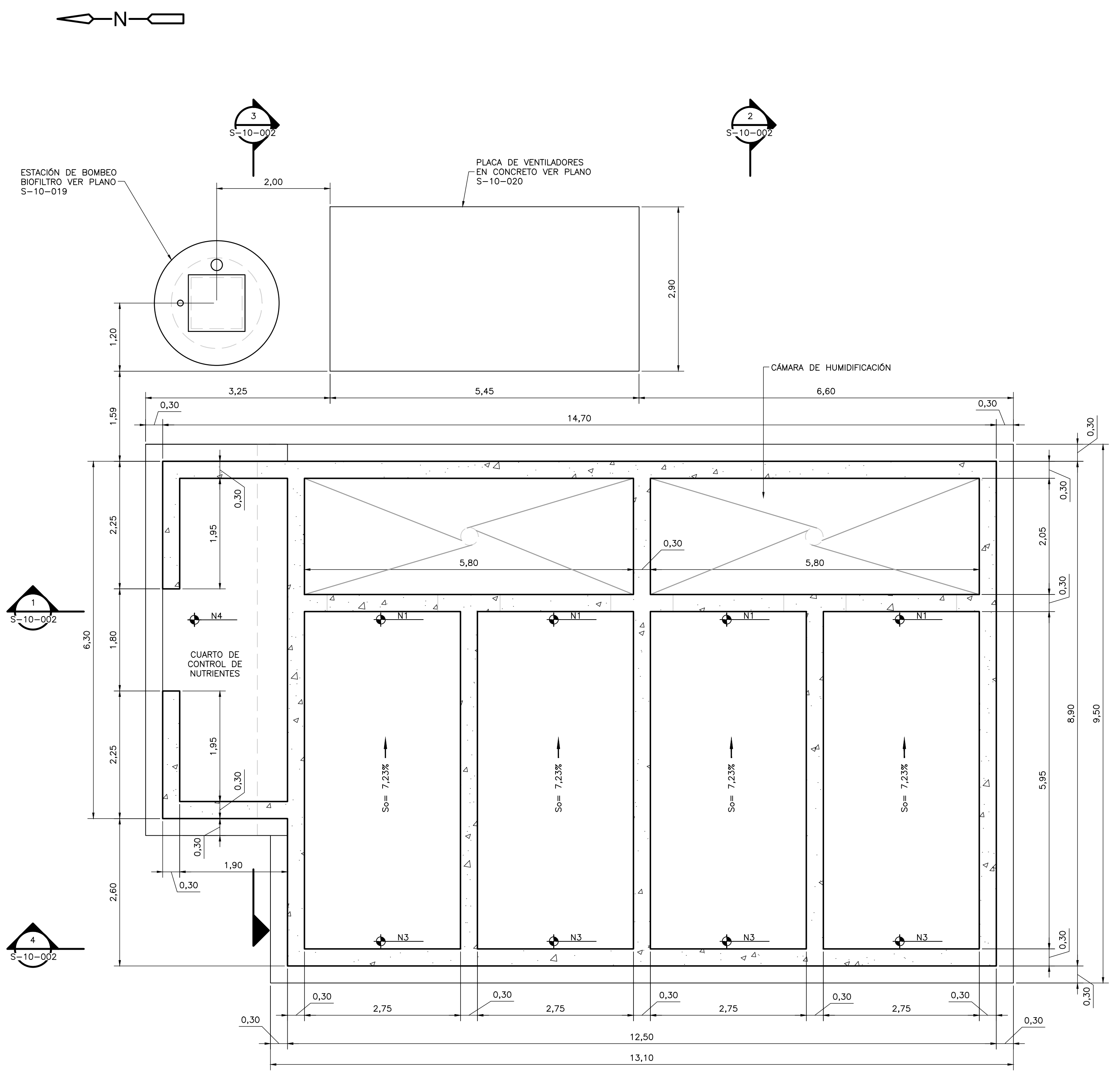
PLANTA INFERIOR 1:50
