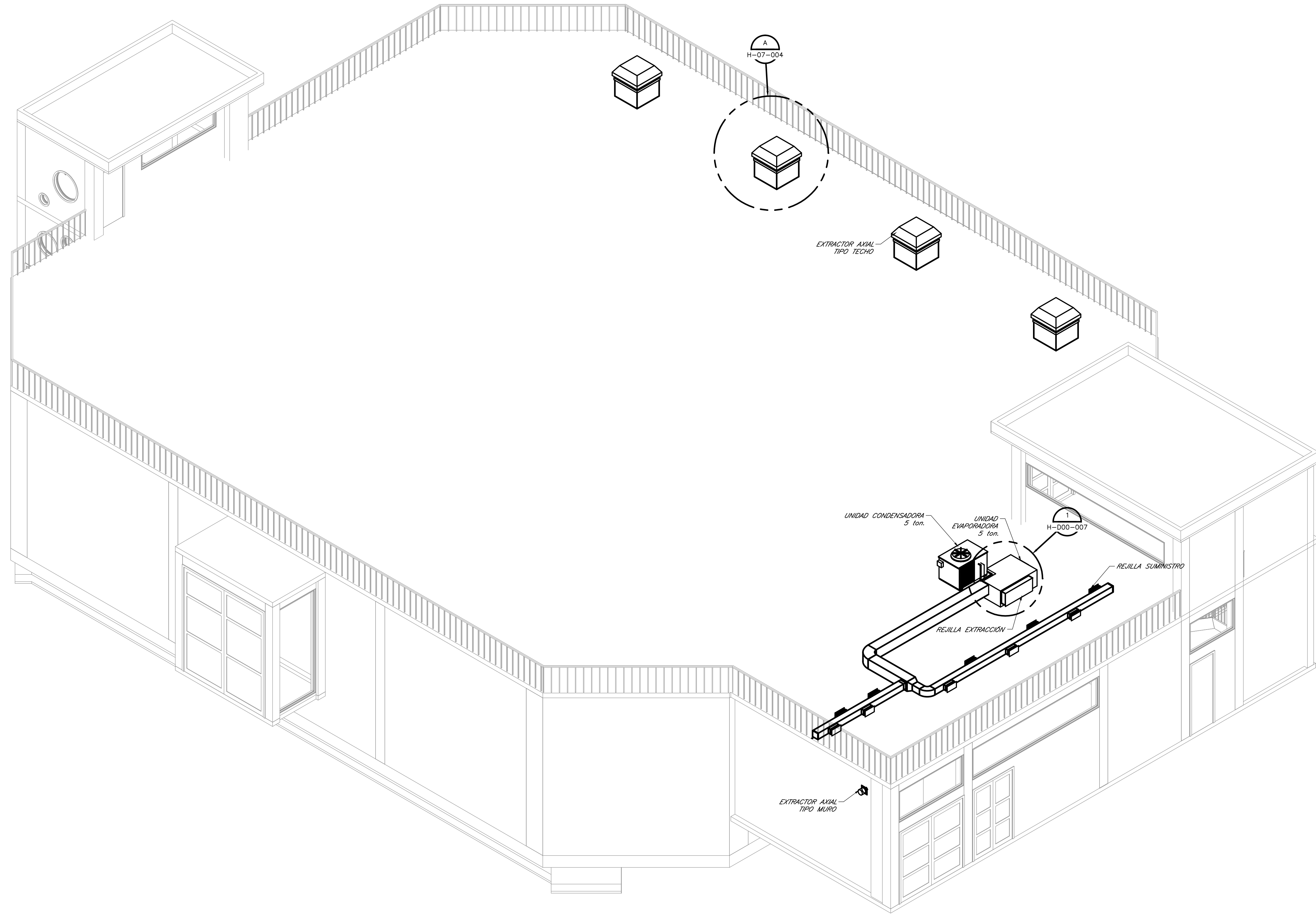
ISOMETRÍA A SIN ESCALA H-07-004
