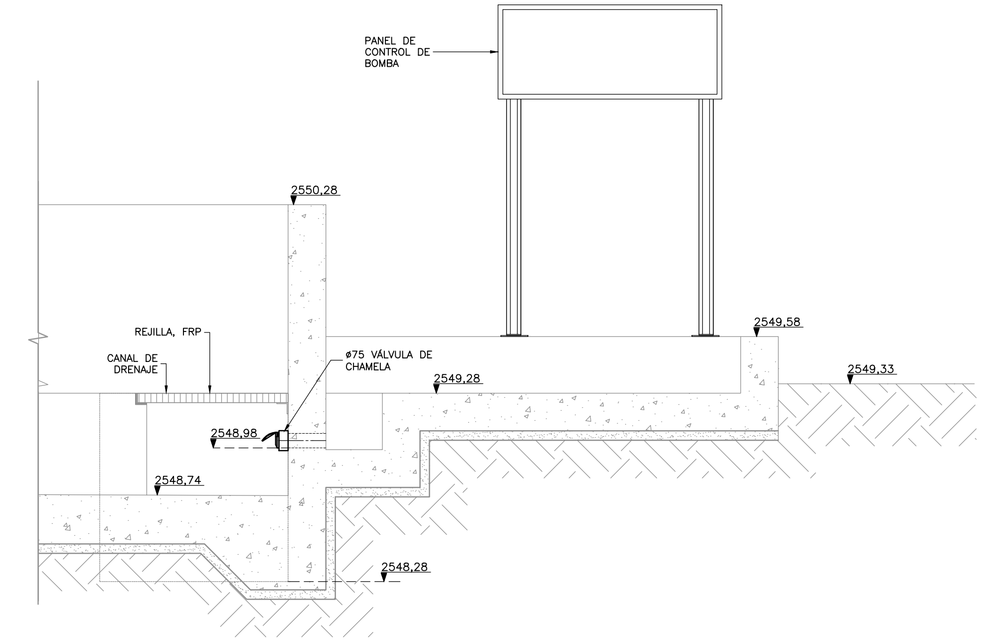
SECCIÓN 4 1=20 M-03-006
