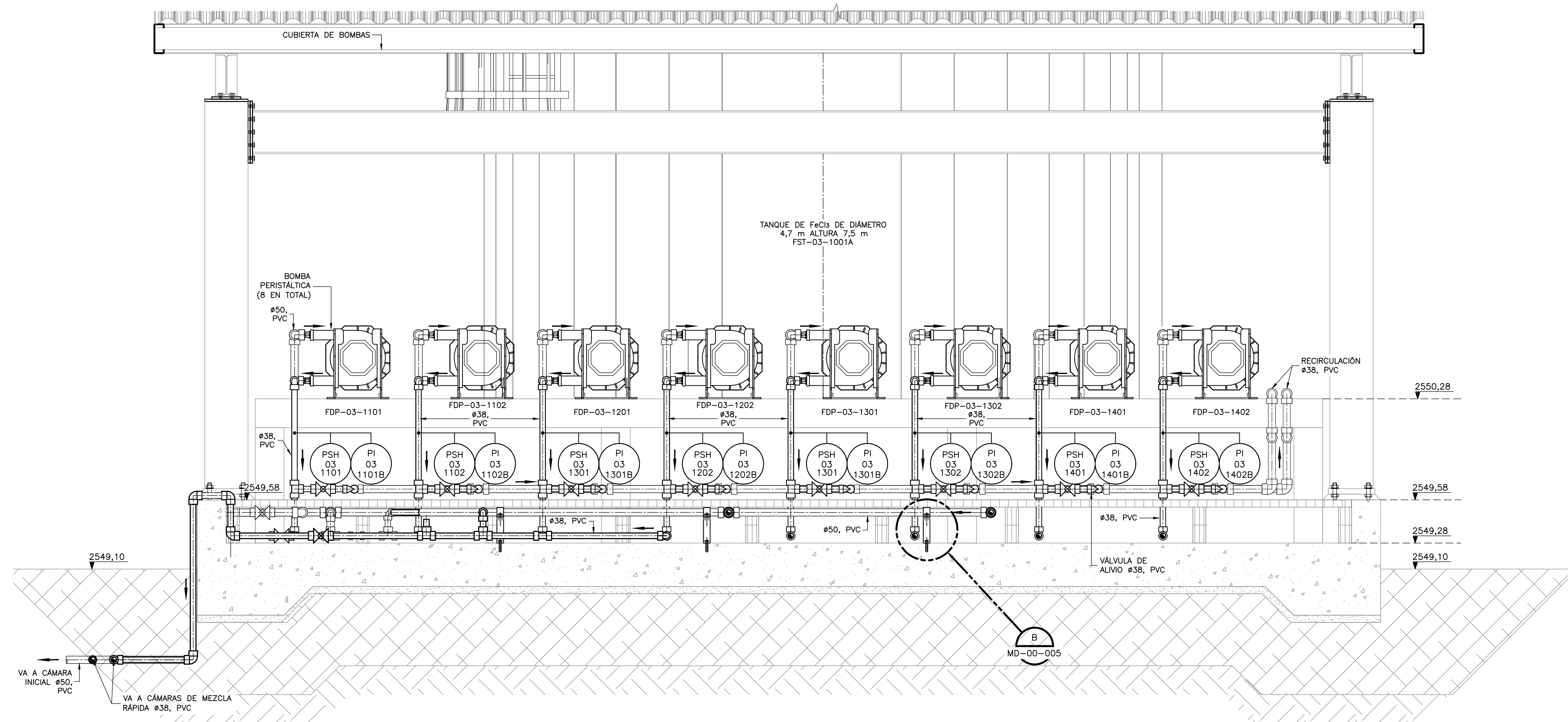
SECCIÓN 3 1=20 M-03-004 M-03-006
