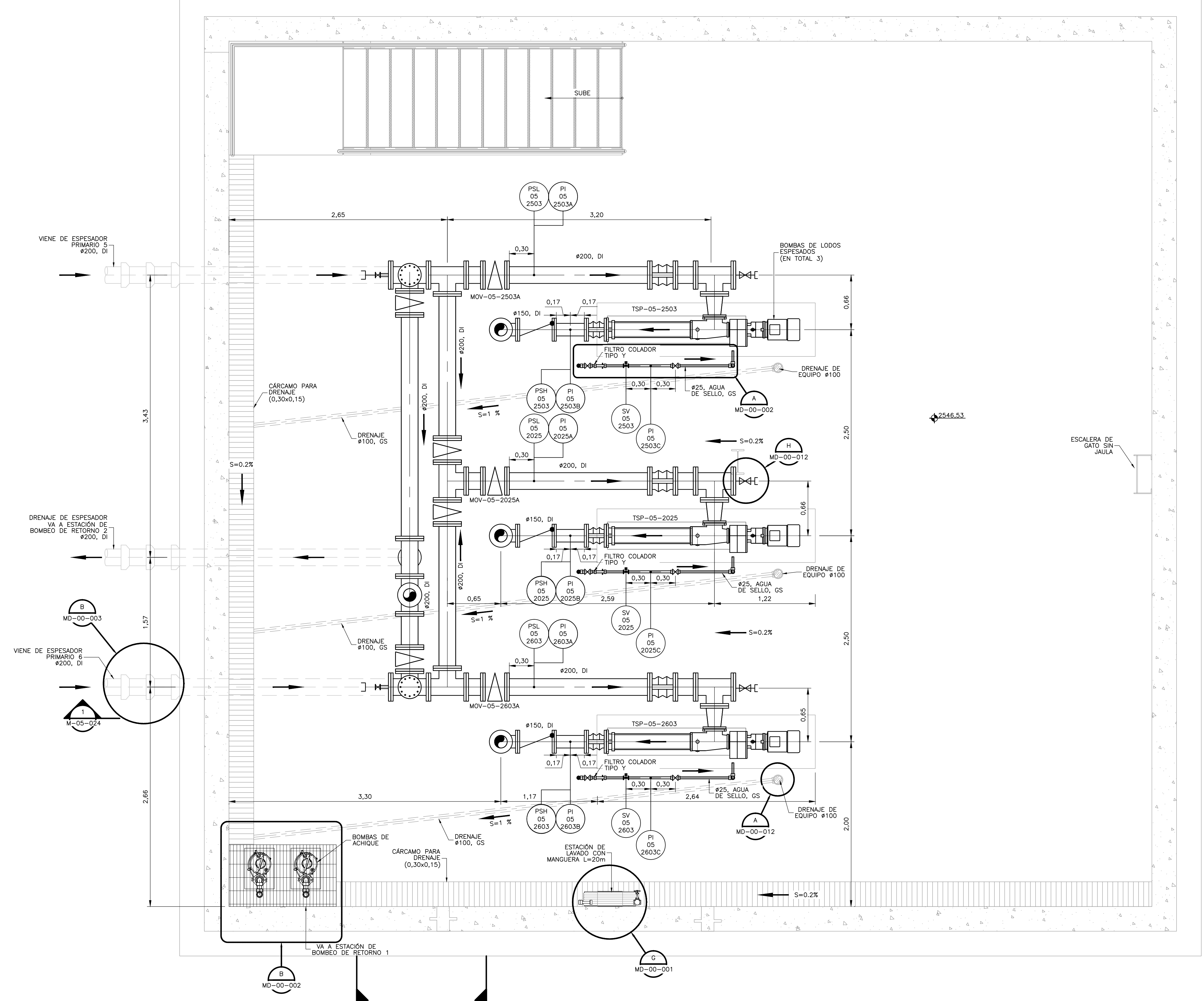
PLANTA INFERIOR 1=25
