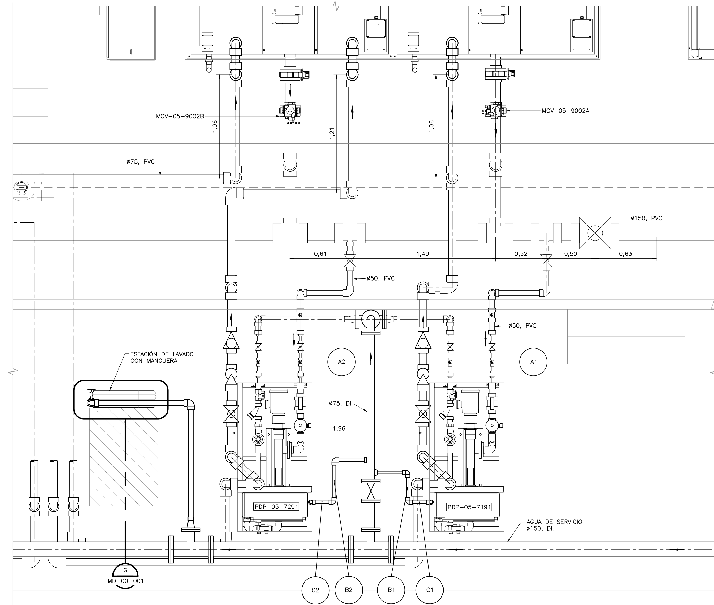
PLANTA POLÍMERO DETALLE F 1=20 M-05-050
