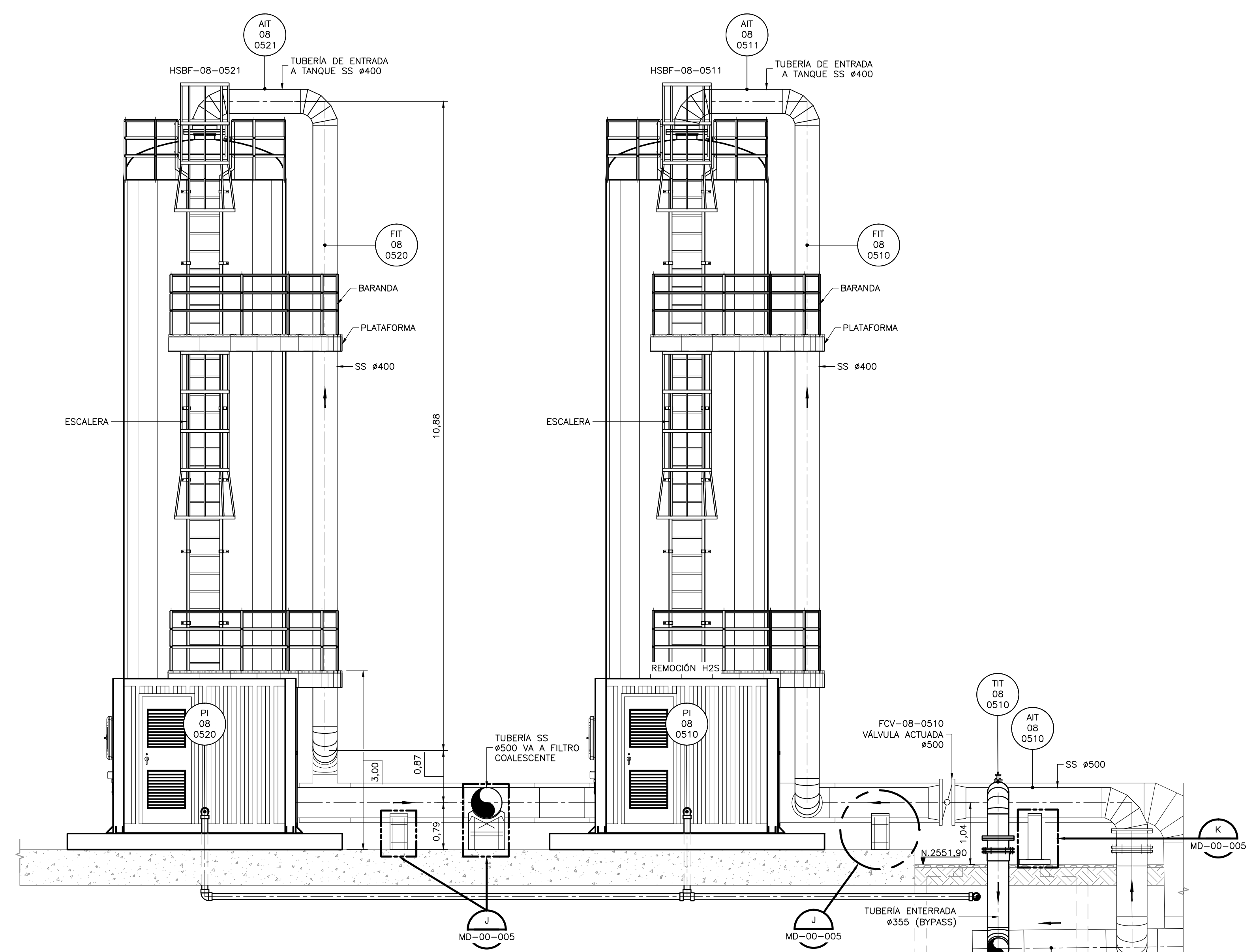
SECCIÓN 3 1=50 M-08-002
