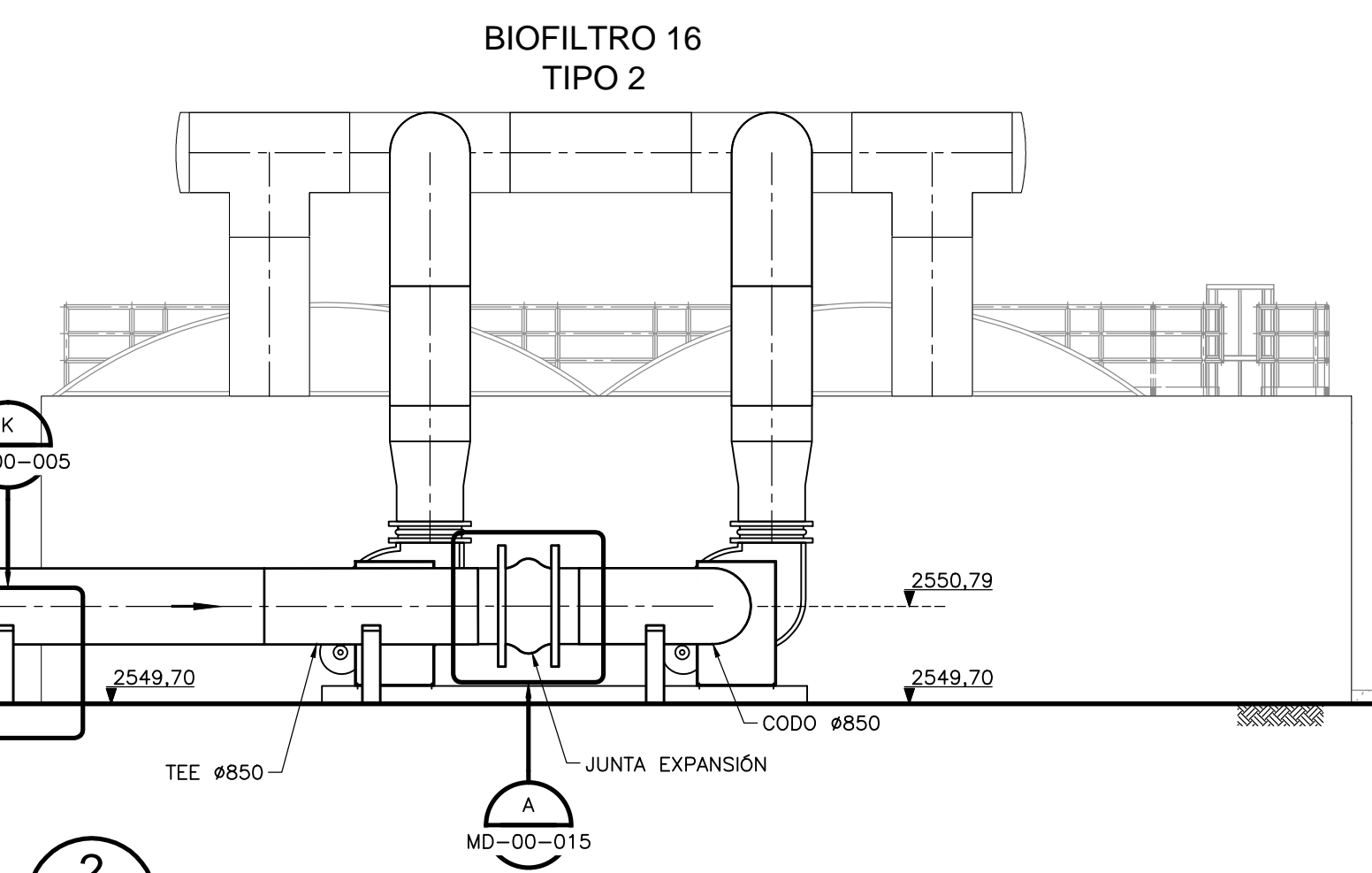
SECCIÓN 2 1=75 M-10-071
