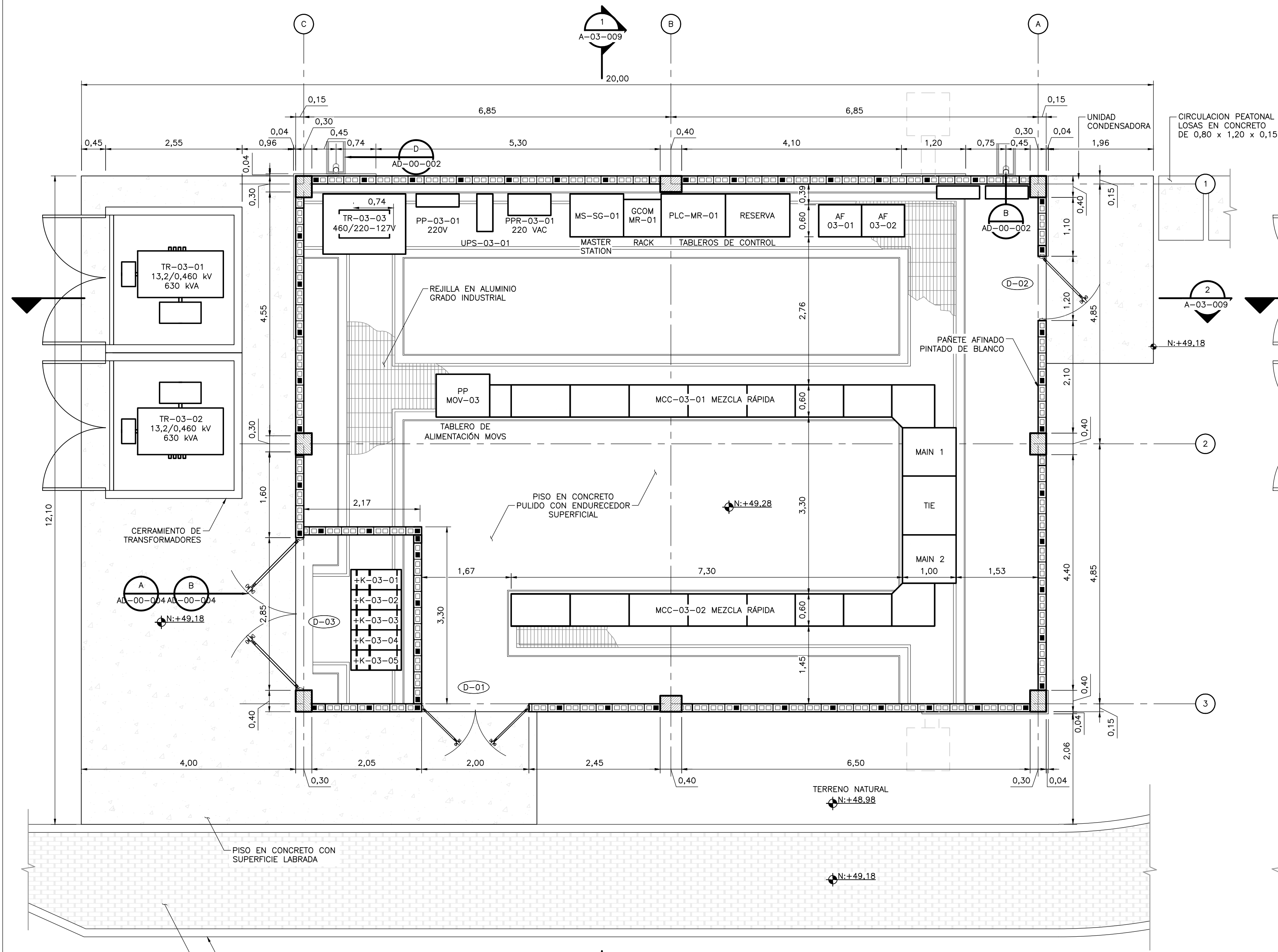
PLANTA PRIMER PISO 1=50
