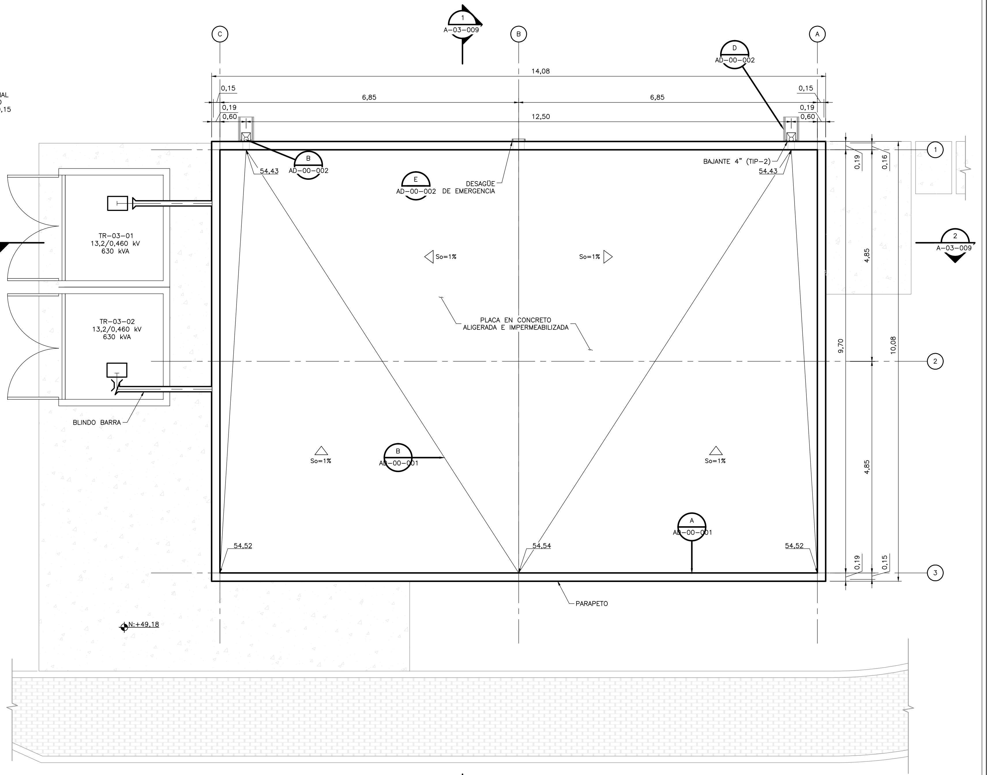
PLANTA CUBIERTA 1=50
