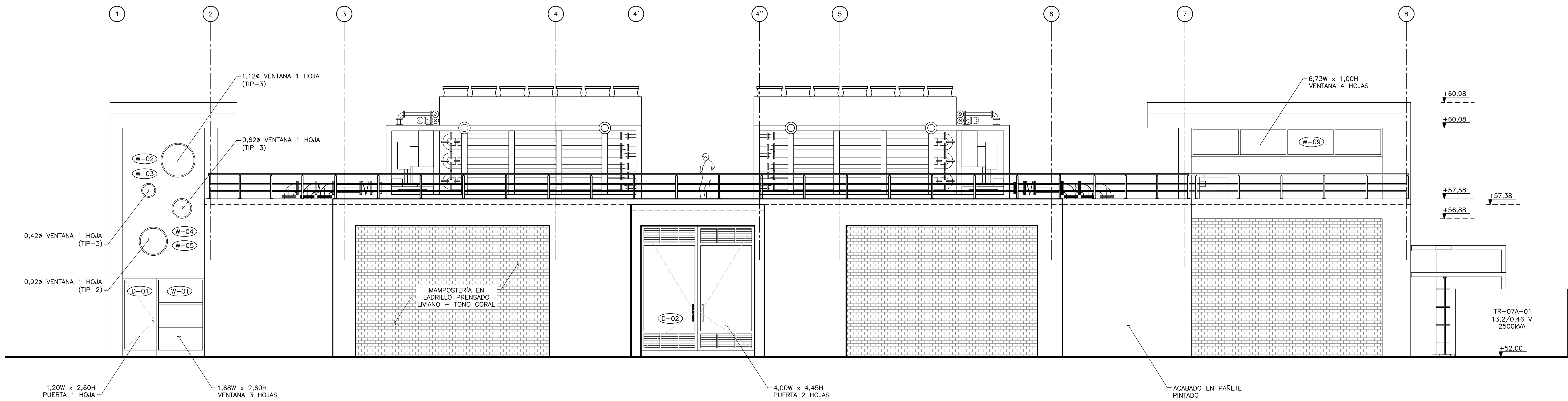
EDIFICIO CONTROL DE DIGESTORES 1 FACHADA OCCIDENTAL 1=75
