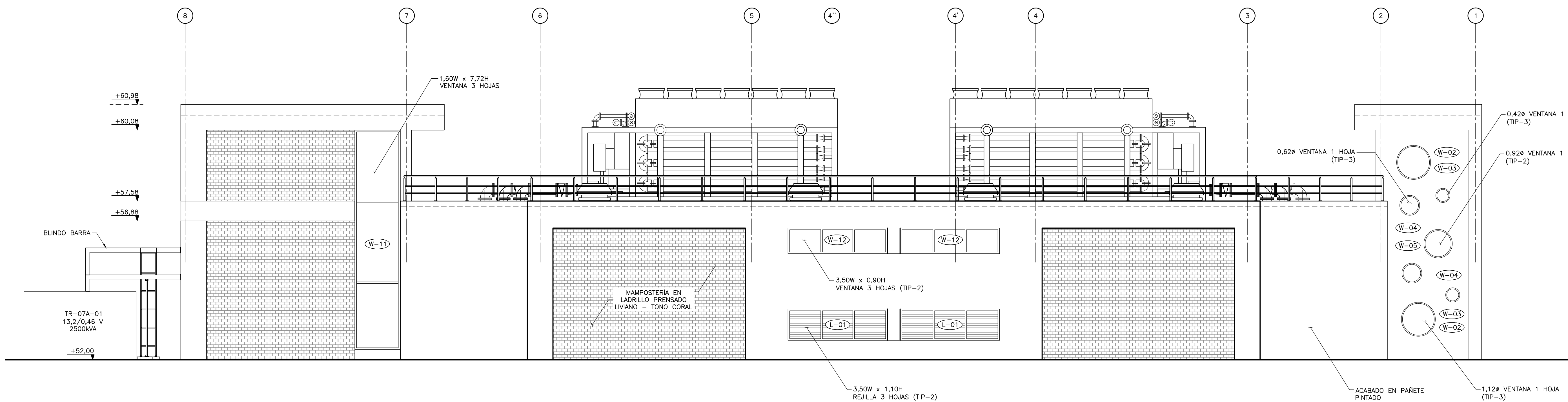
EDIFICIO CONTROL DE DIGESTORES 1 FACHADA ORIENTAL 1=75
