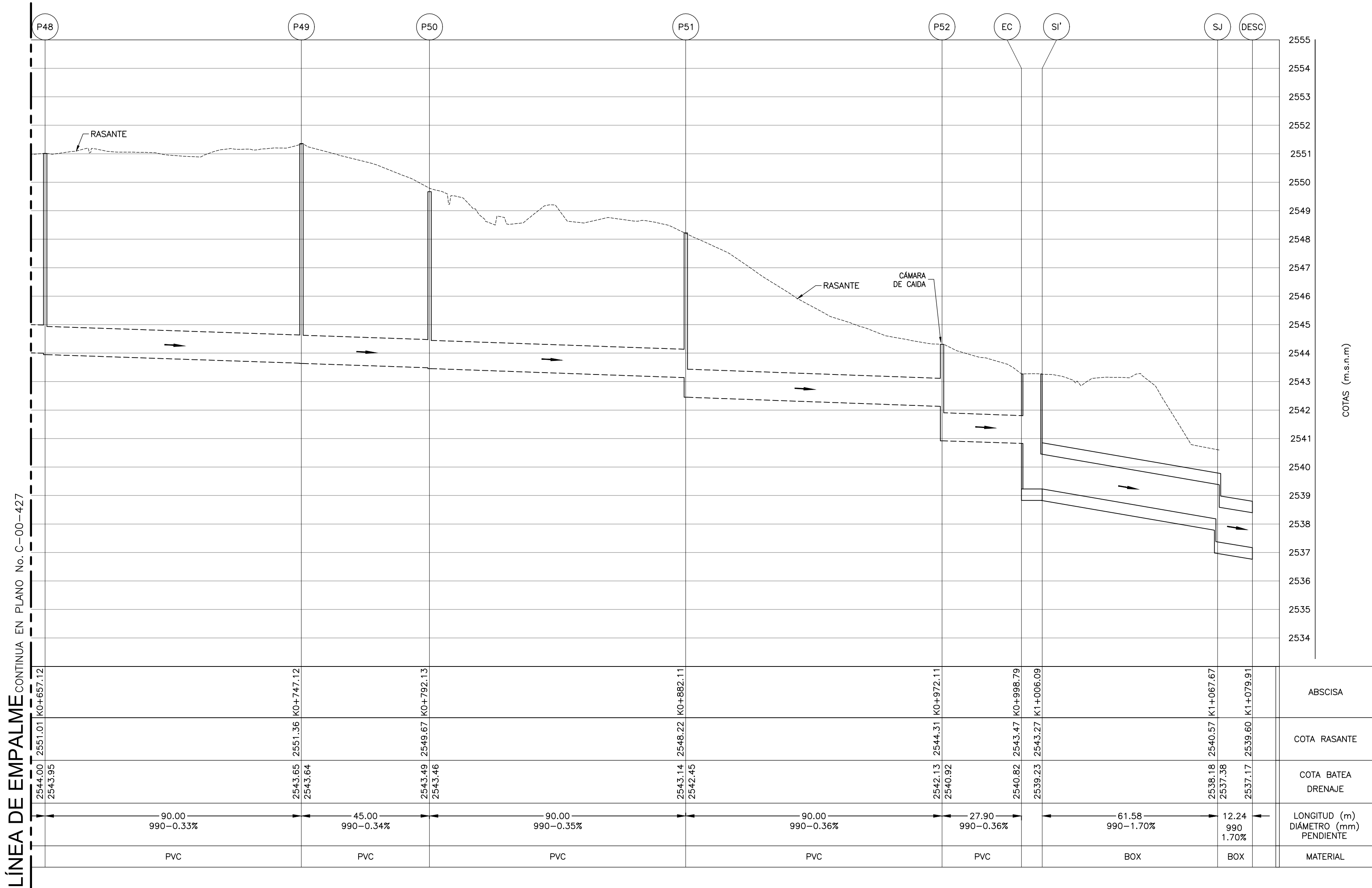
PERFIL LONGITUDINAL P48 A DESCARGA ESCALA H = 100 - V = 1000
