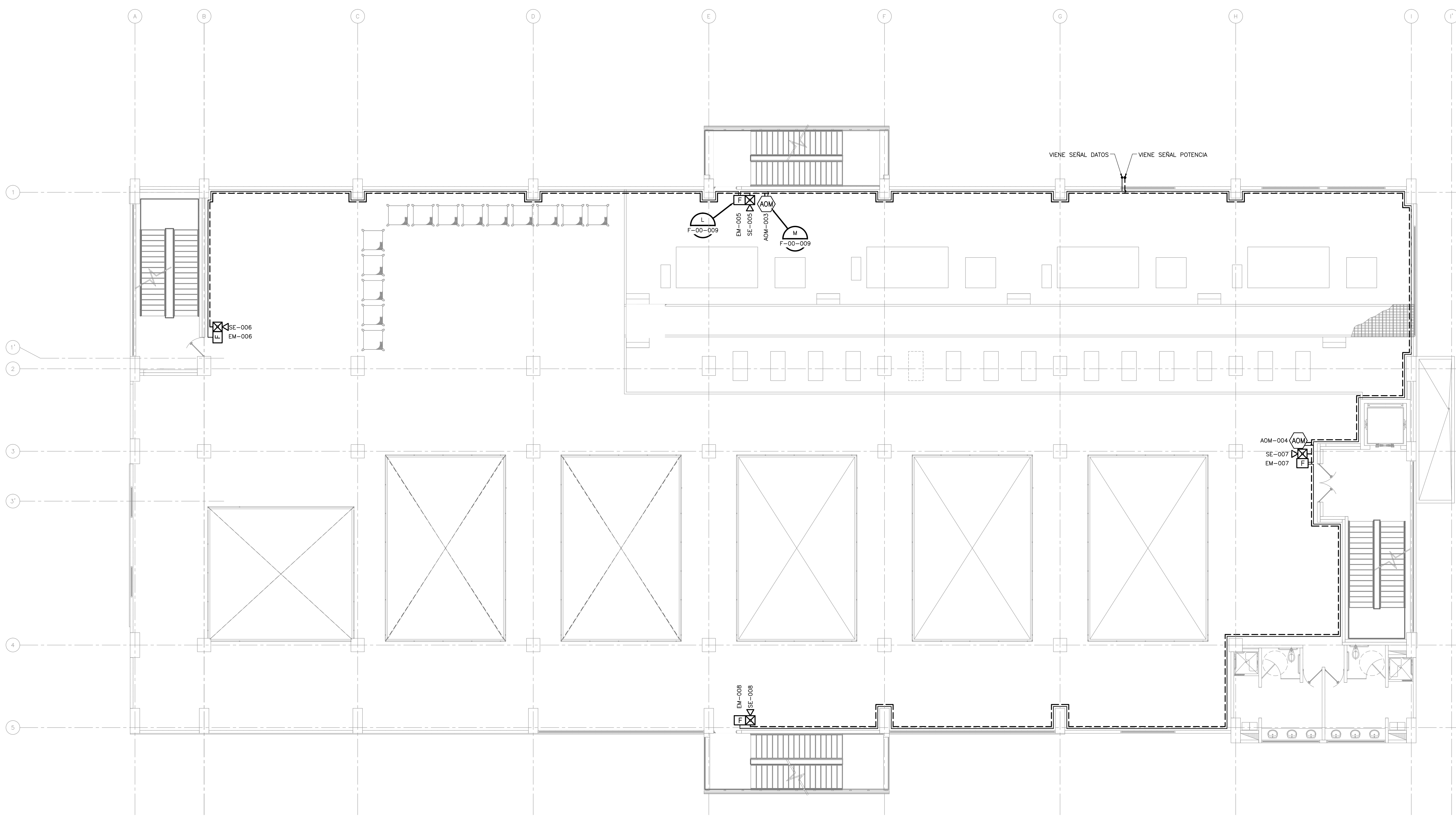
PLANTA 1=100
