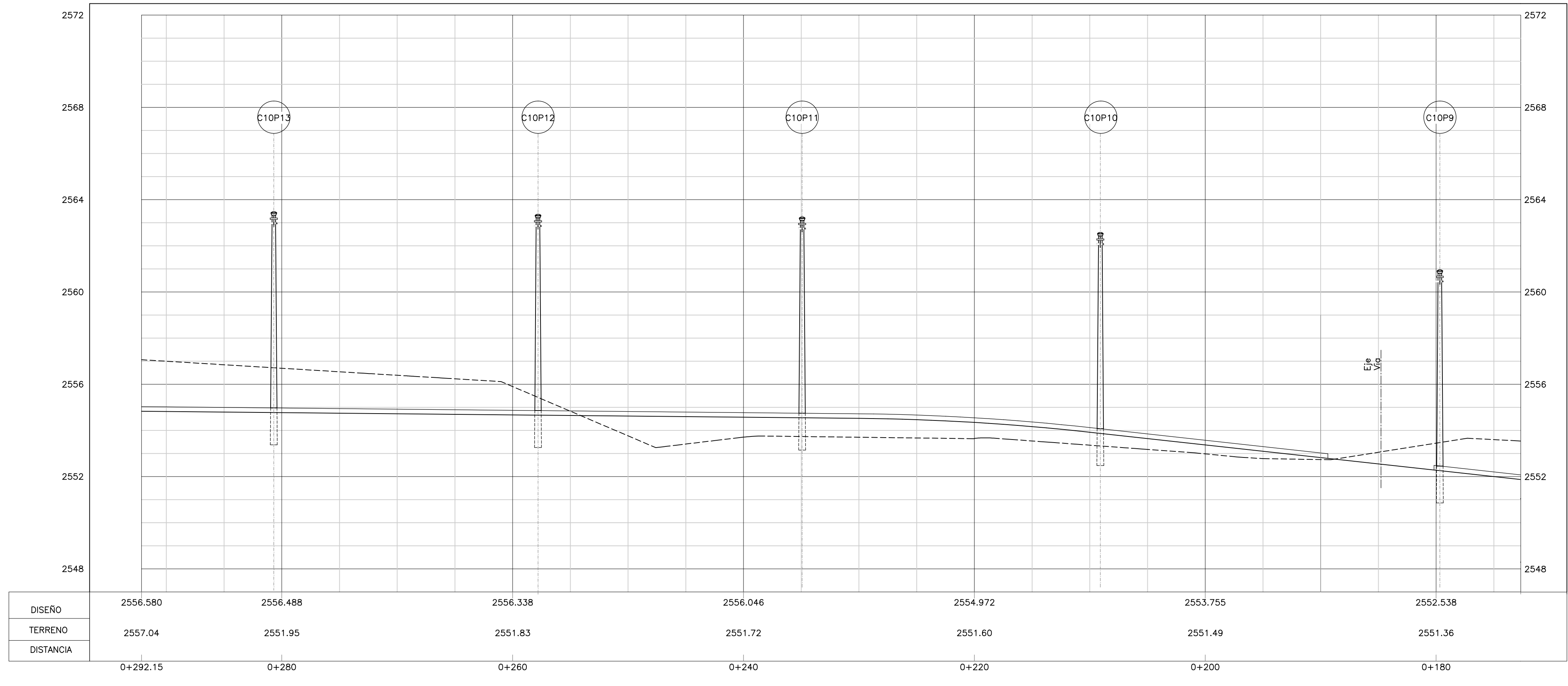
PERFIL 3 H:1:250 V:1:125 E-00-032
