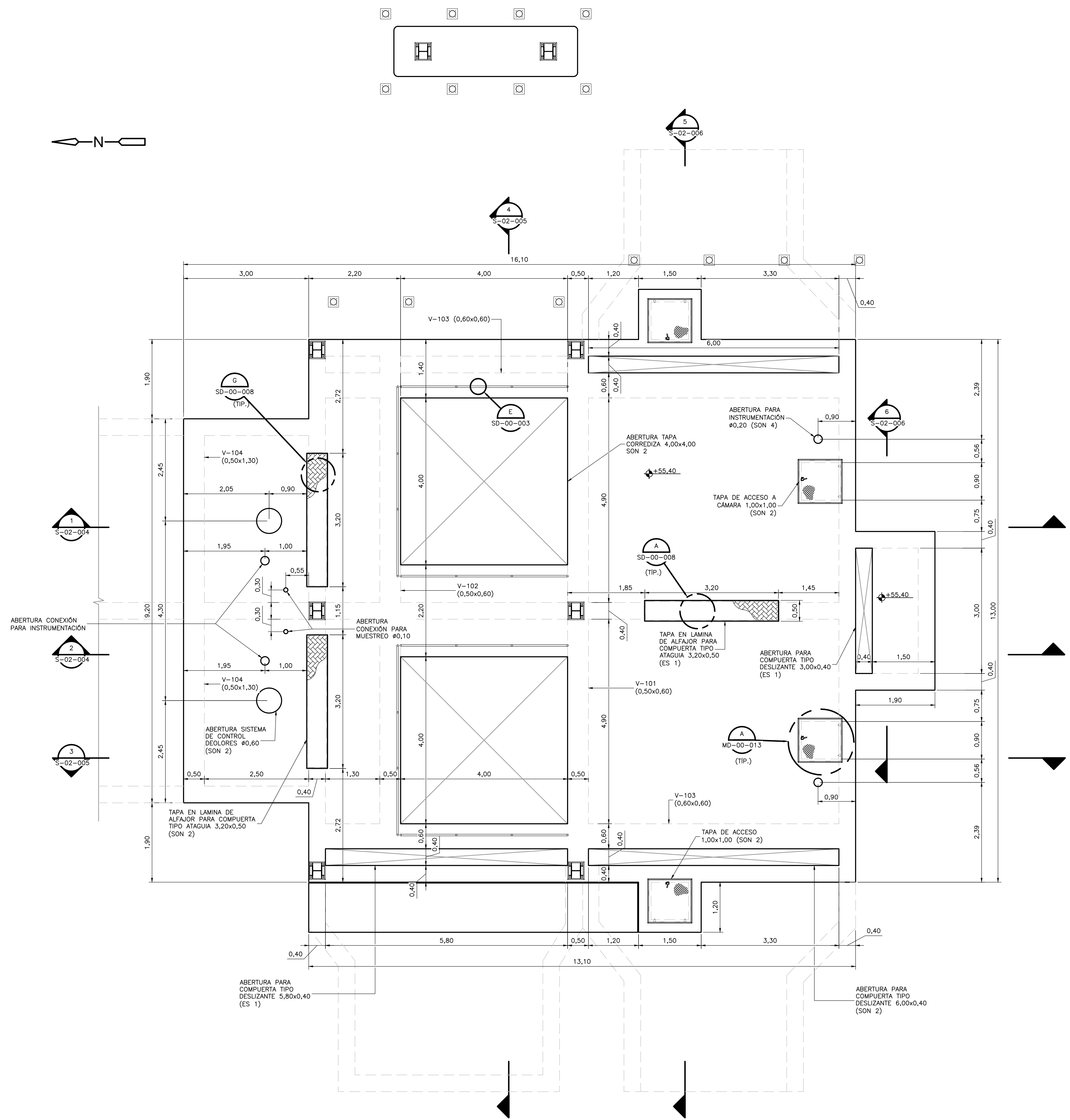
PLANTA SUPERIOR 1=50
