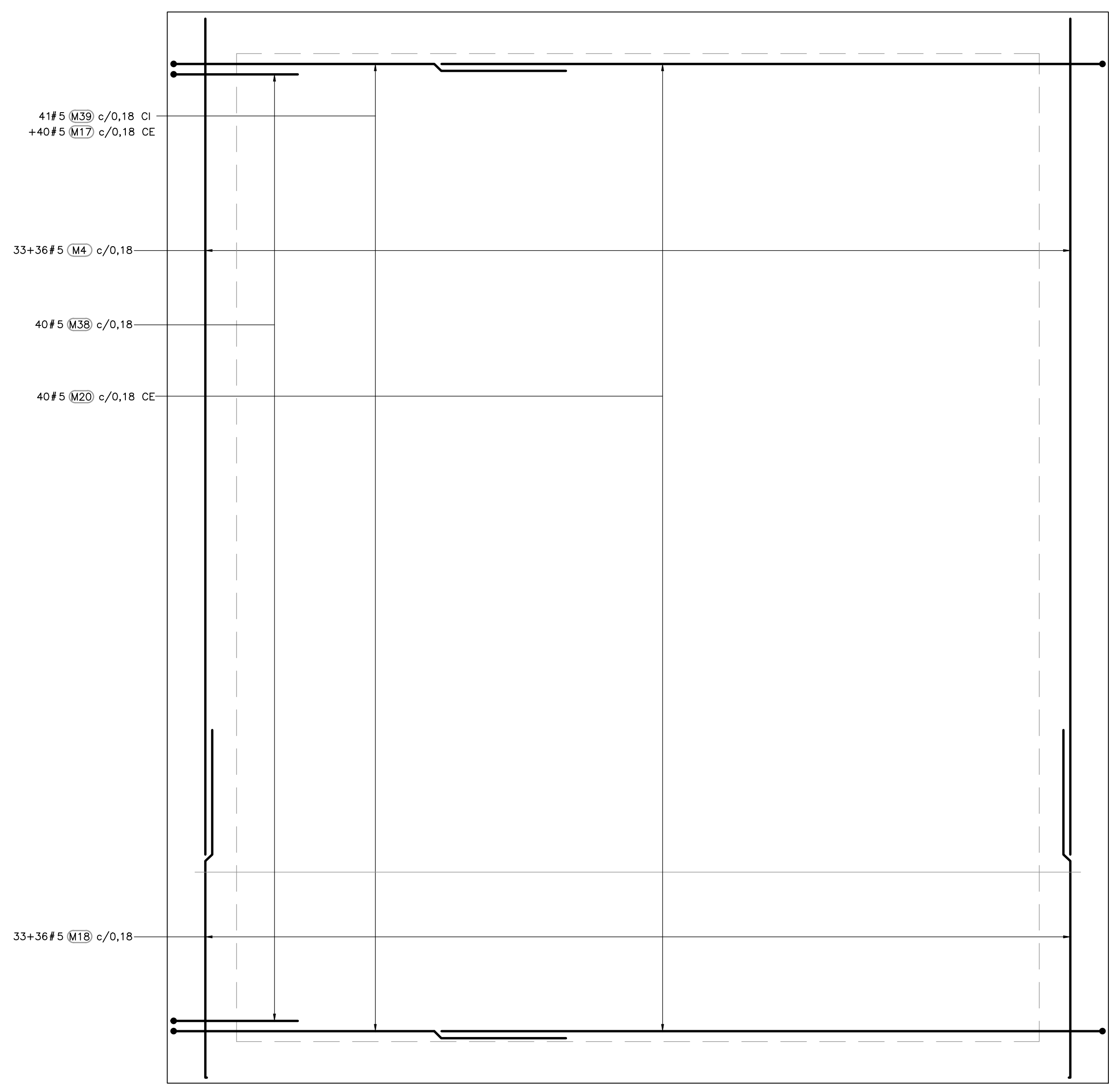
AMBAS CARAS REFUERZO MURO 3 (SON 2) 1=25
