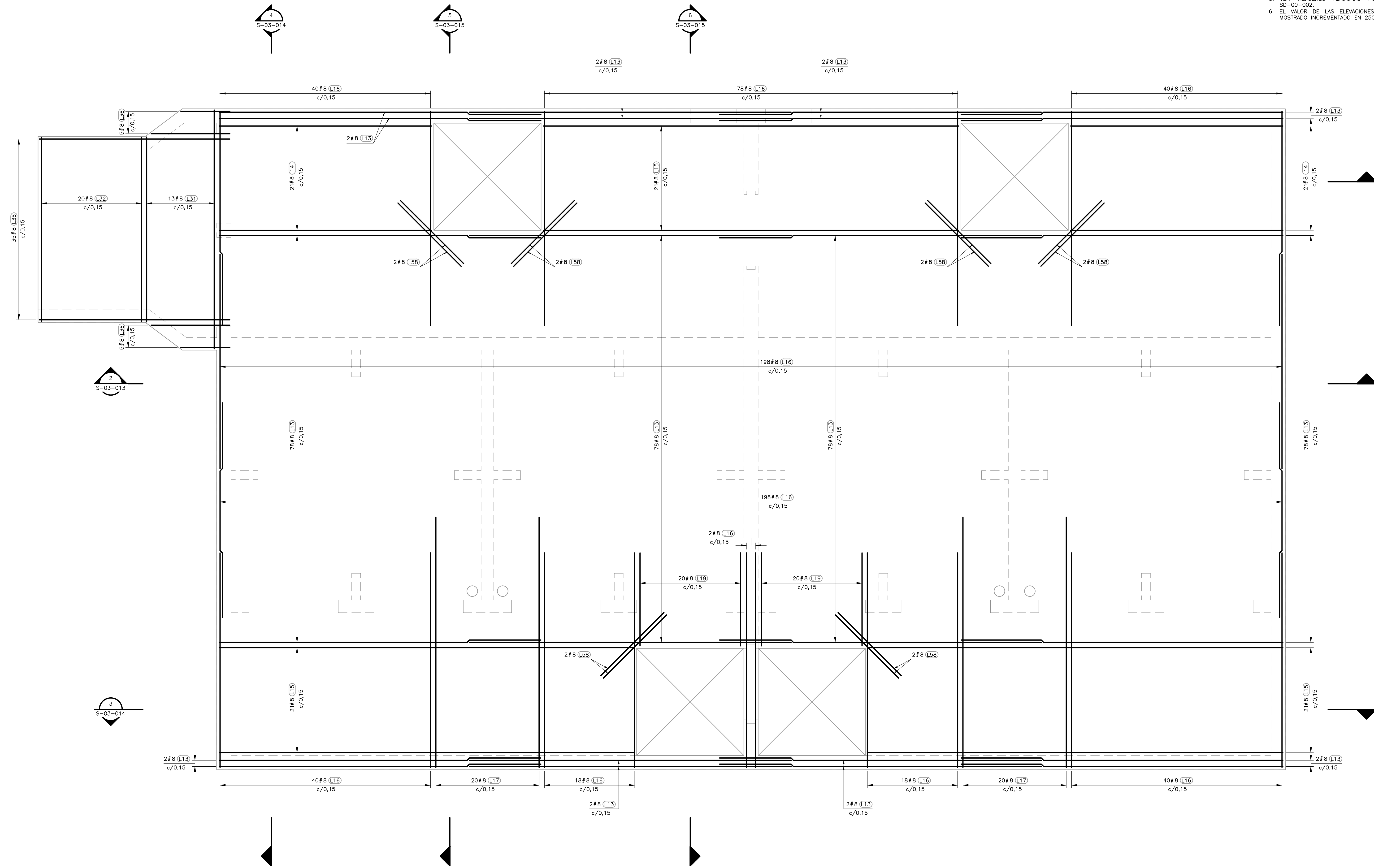
REFUERZO INFERIOR PLANTA LOSA INFERIOR NIVEL: 2547,18 1=50
