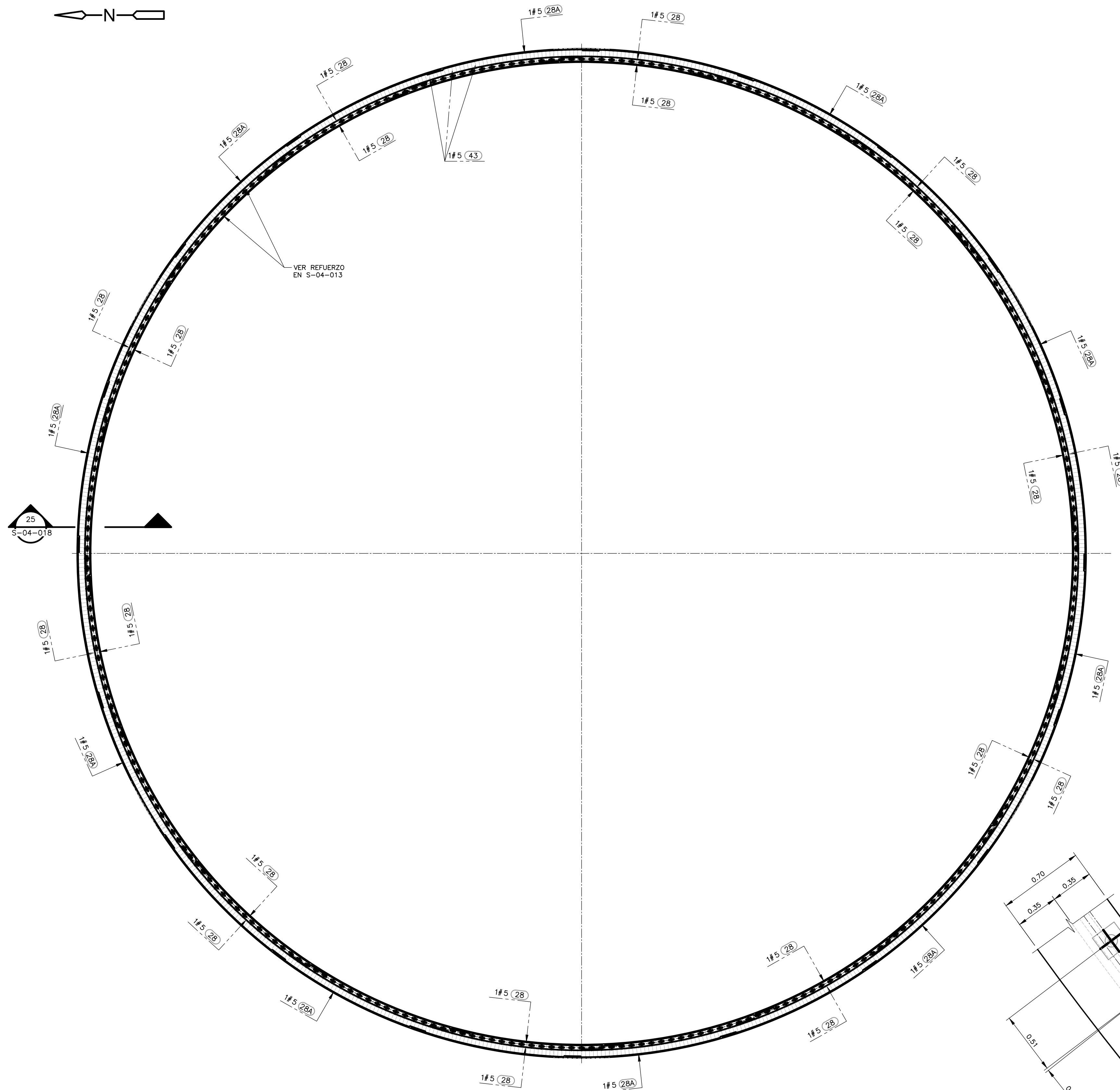
LOCALIZACION REFUERZO PLANTA VIGA BORDE DE CUBIERTA 1 = 125
