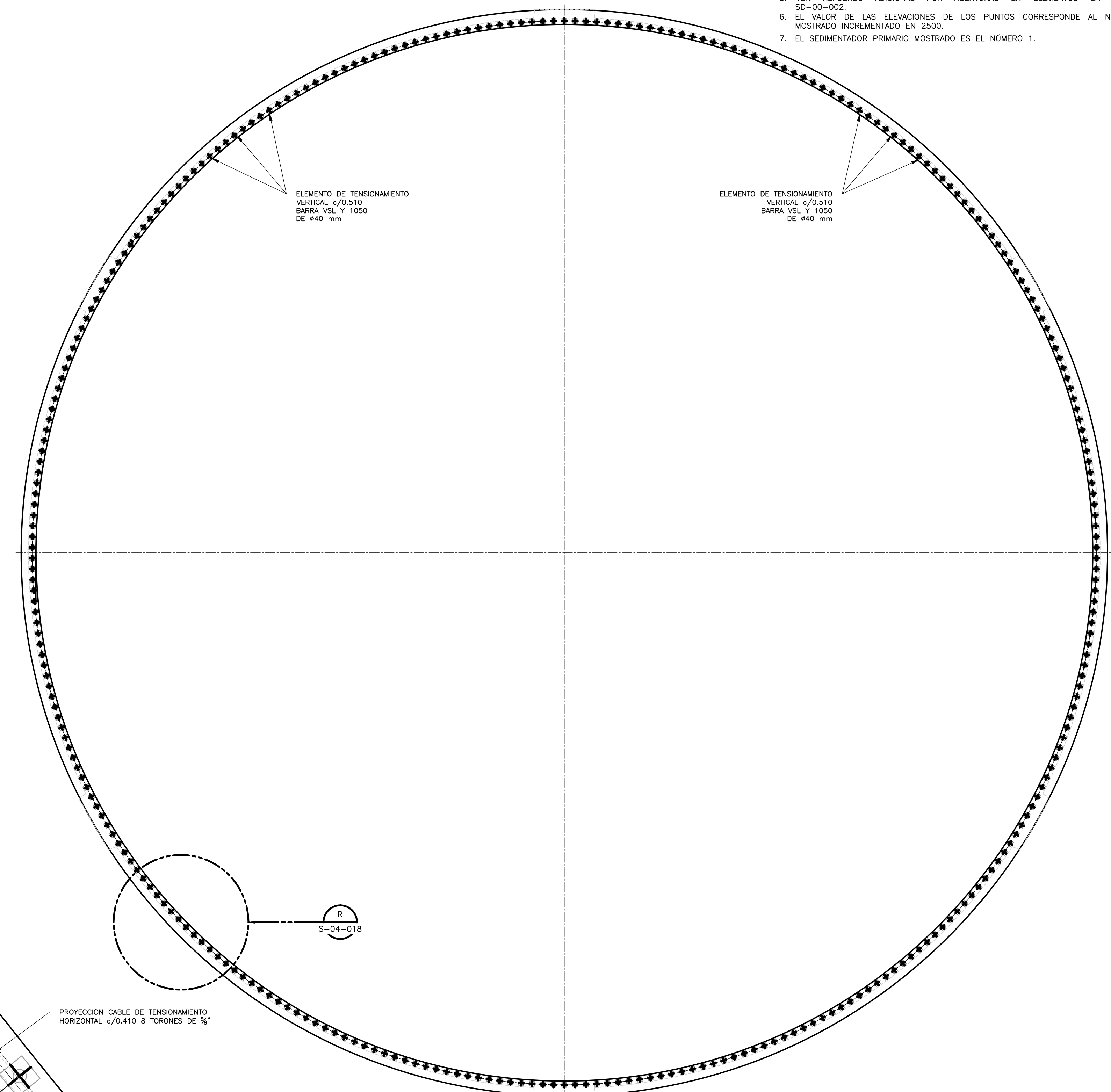
LOCALIZACIÓN CABLES DE TENSIONAMIENTO VERTICAL PLANTA DE CUBIERTA 1 = 125
