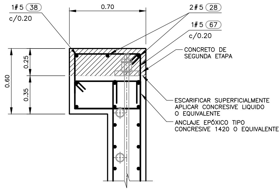
SECCION VIGA 25 1=20 S-04-018
