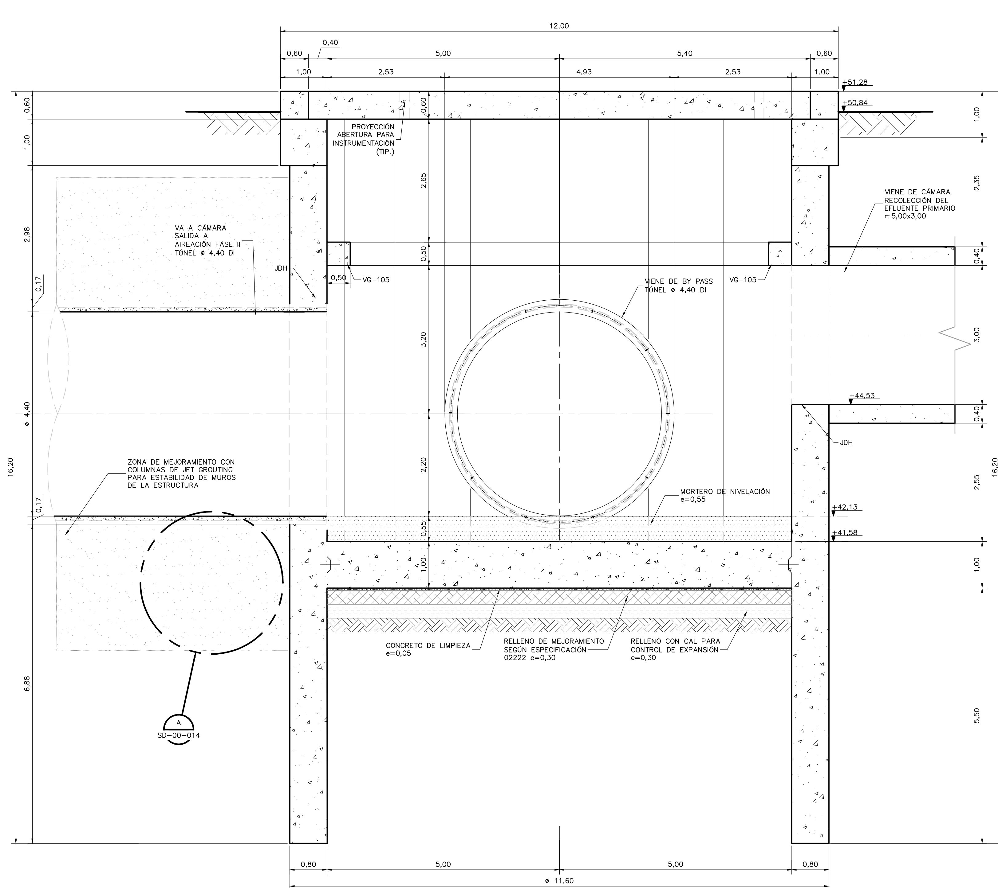
SECCIÓN 1 1=50 S-04-033
