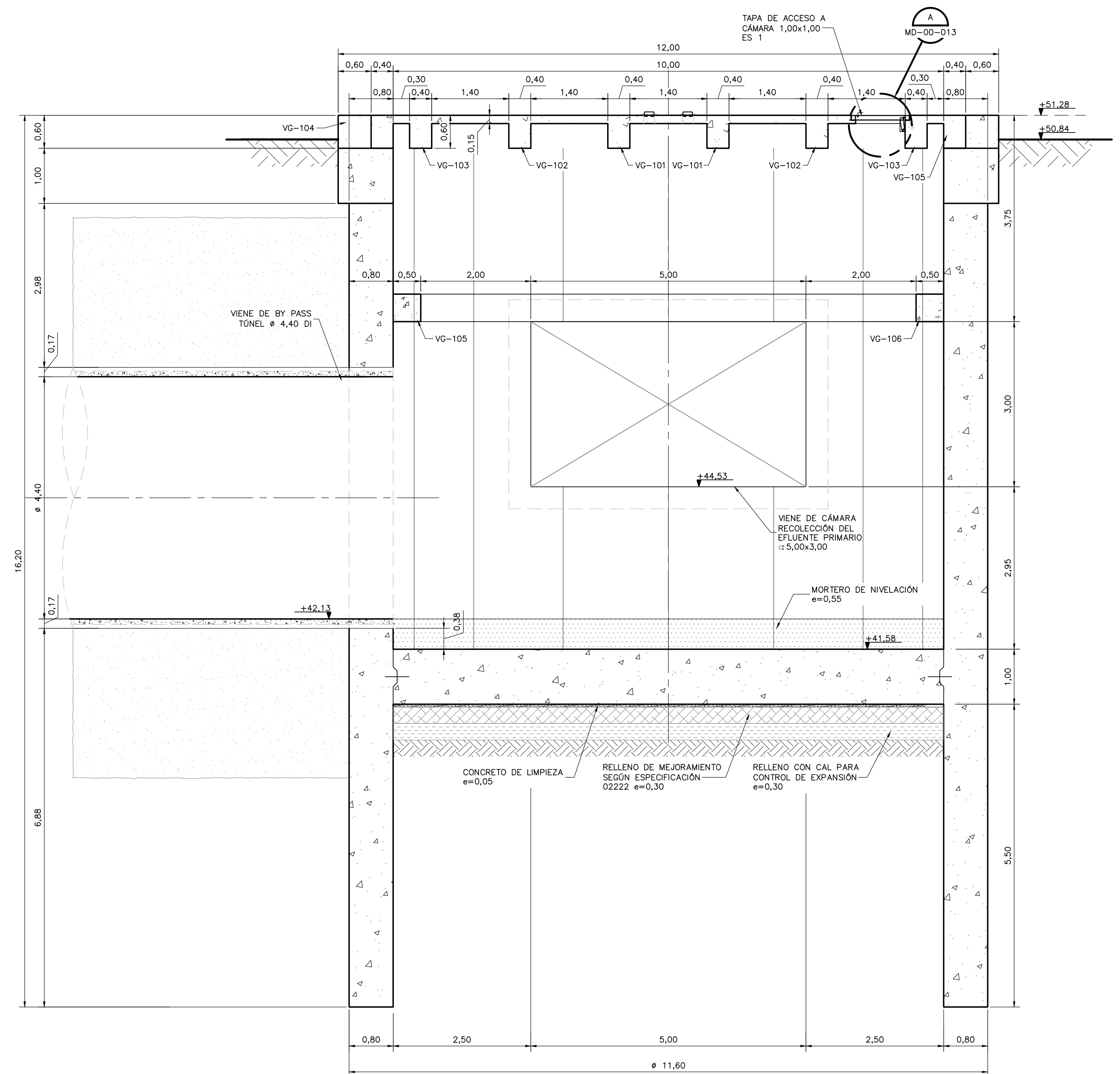
SECCIÓN 2 1=50 S-04-033
