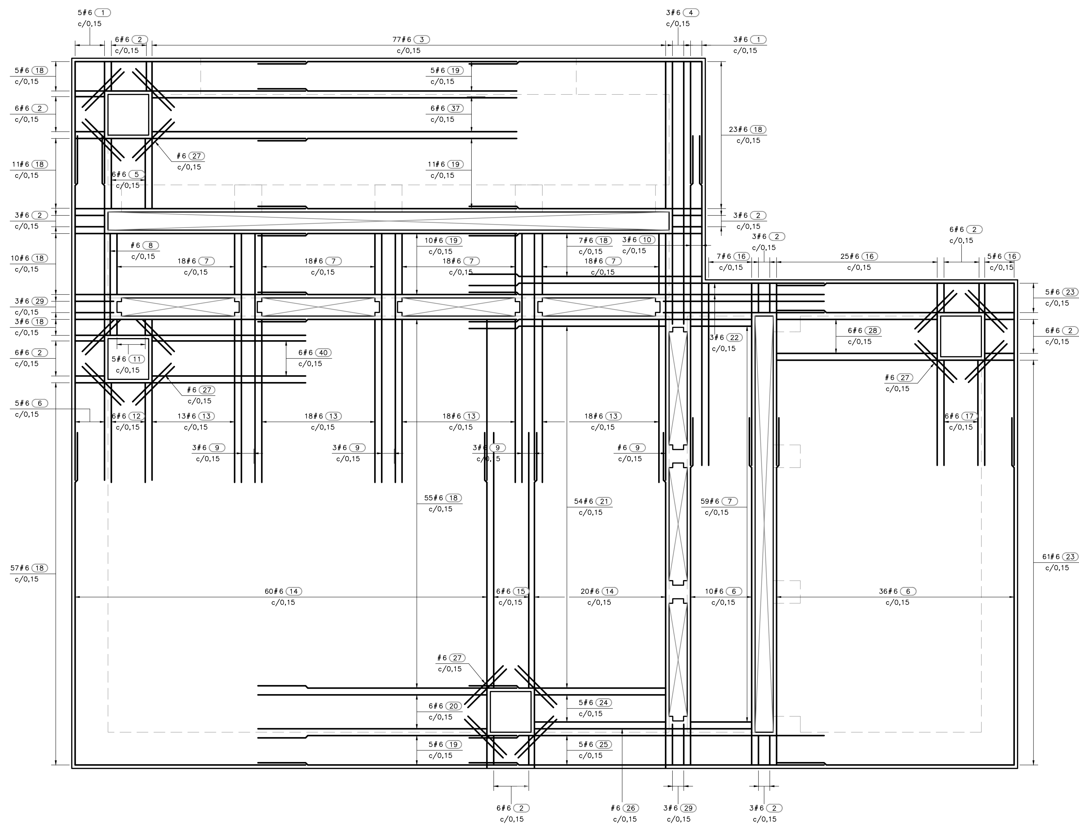
REFUERZO INFERIOR PLACA DE CUBIERTA 1=50
