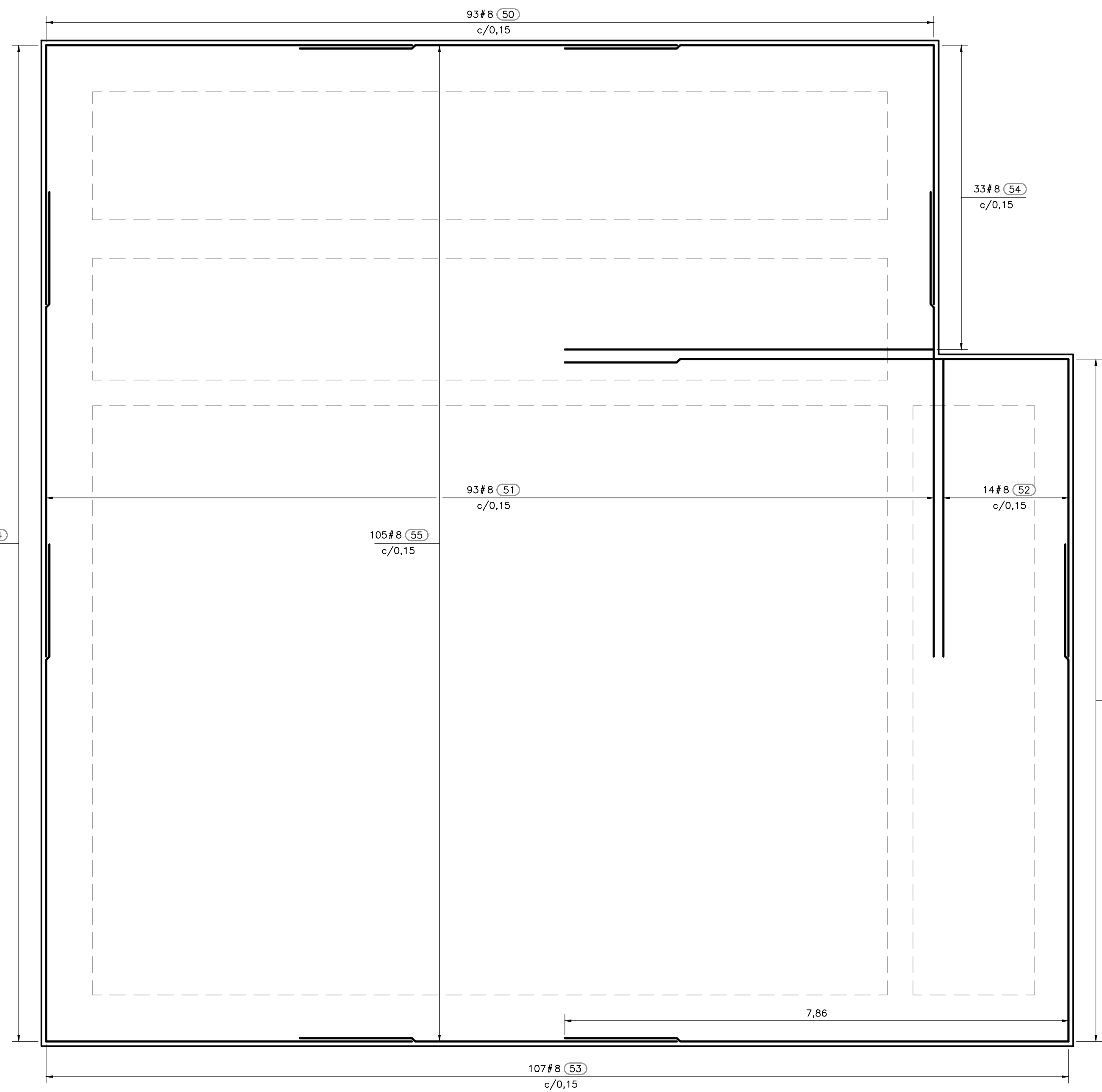
REFUERZO SUPERIOR PLACA NIVEL +41,50 1=50
