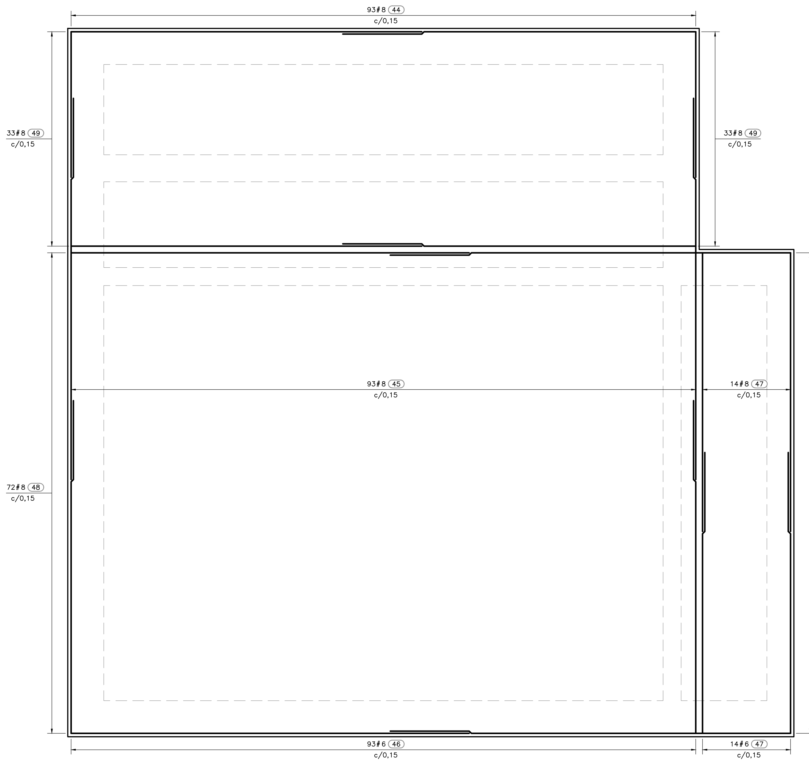
REFUERZO INFERIOR PLACA NIVEL +41,50 1=50
