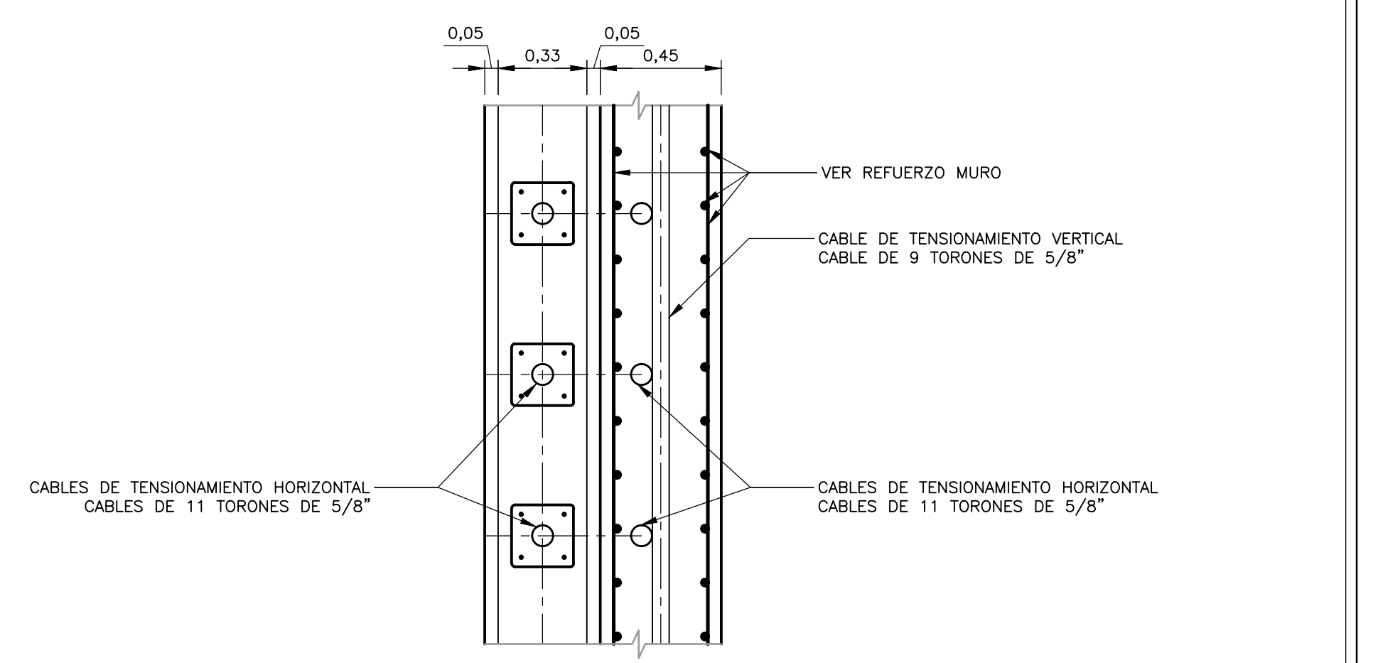
ALZADO CABLES DE TENSIONAMIENTO VERTICAL SECCIÓN C 1=20
