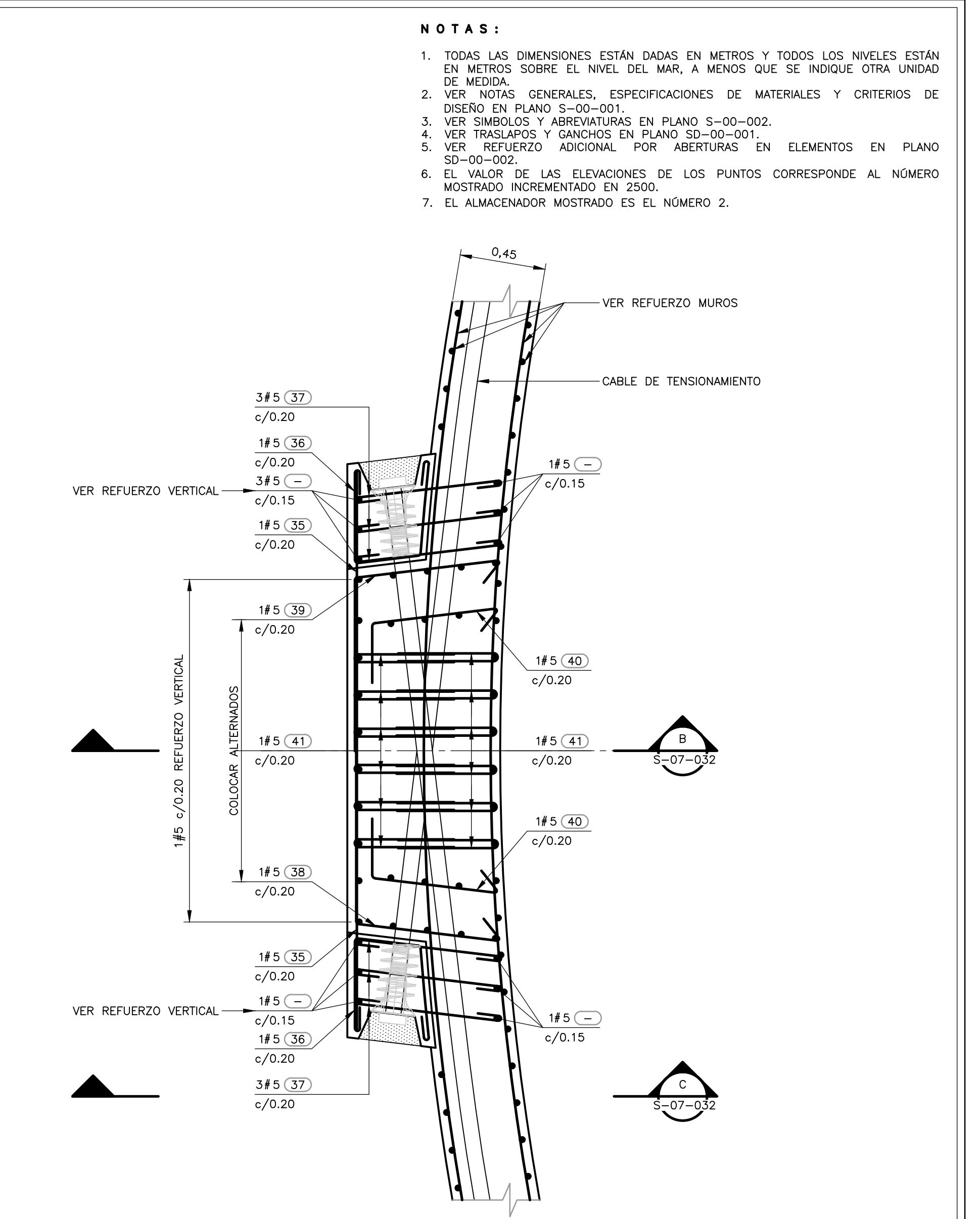
DETALLE 14 REFUERZO COLUMNA DE TENSIONAMIENTO 1=20
