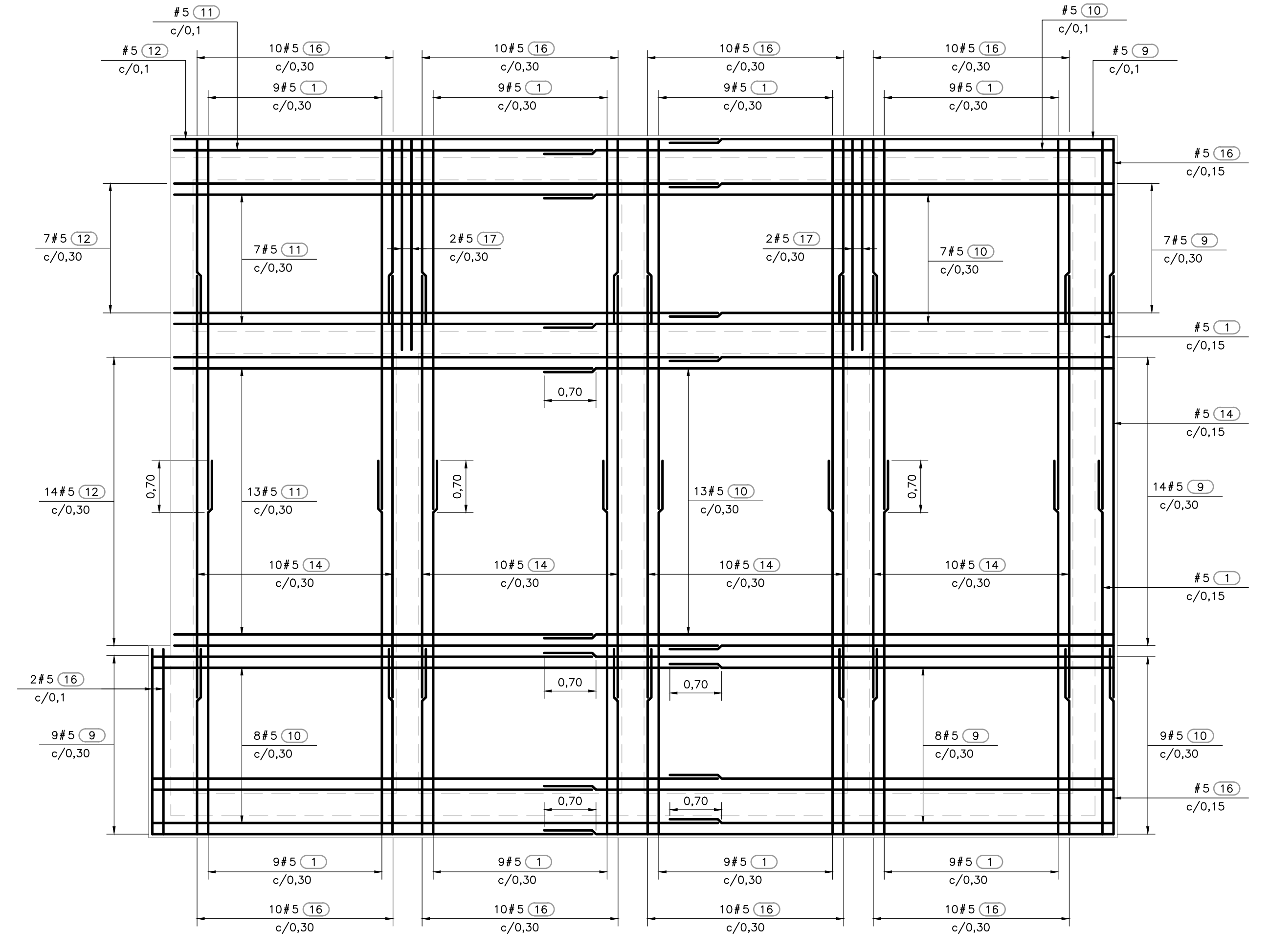
REFUERZO SUPERIOR PLACA DE FONDO 1=50
