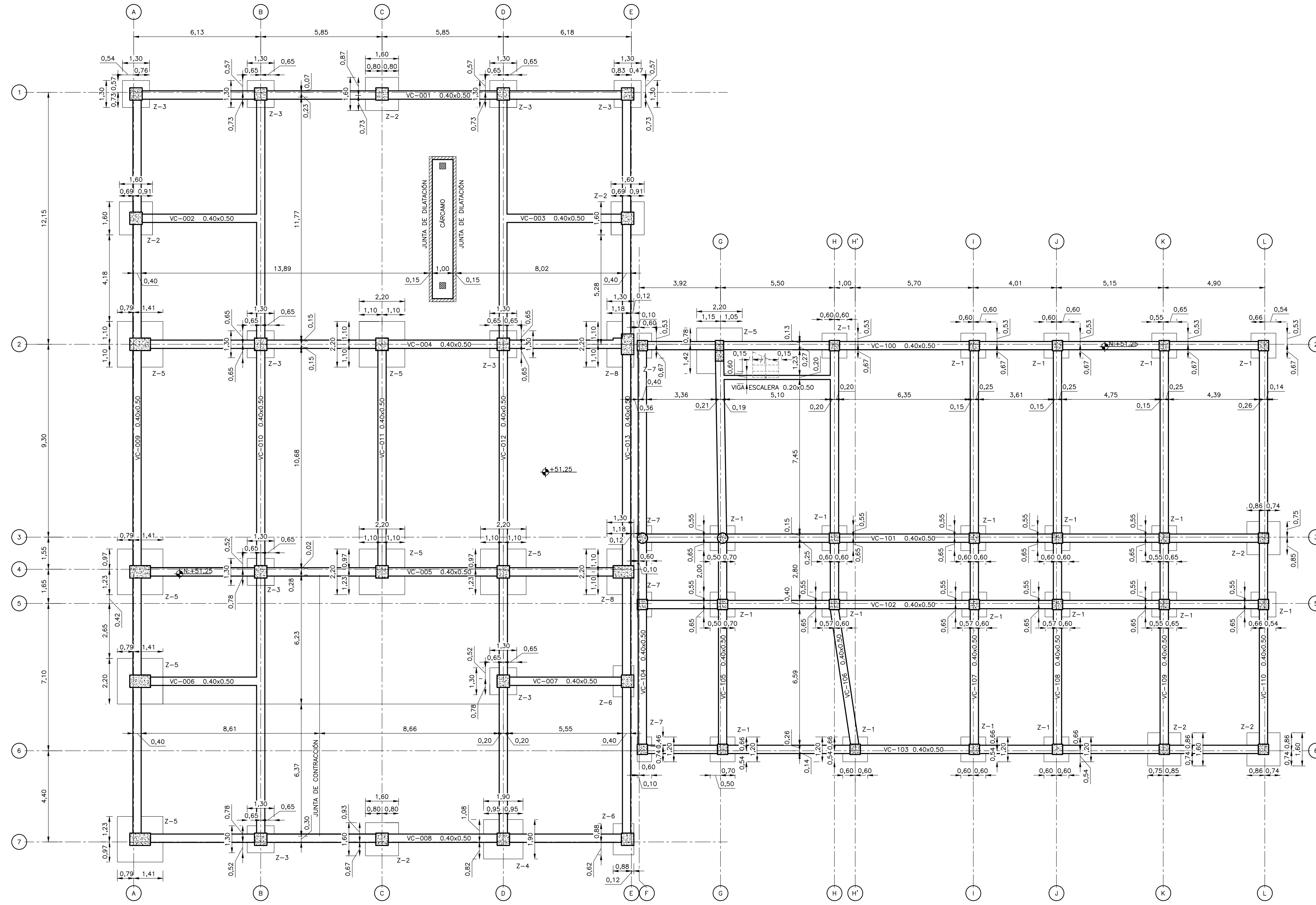
PLANTA DE CIMENTACIÓN
