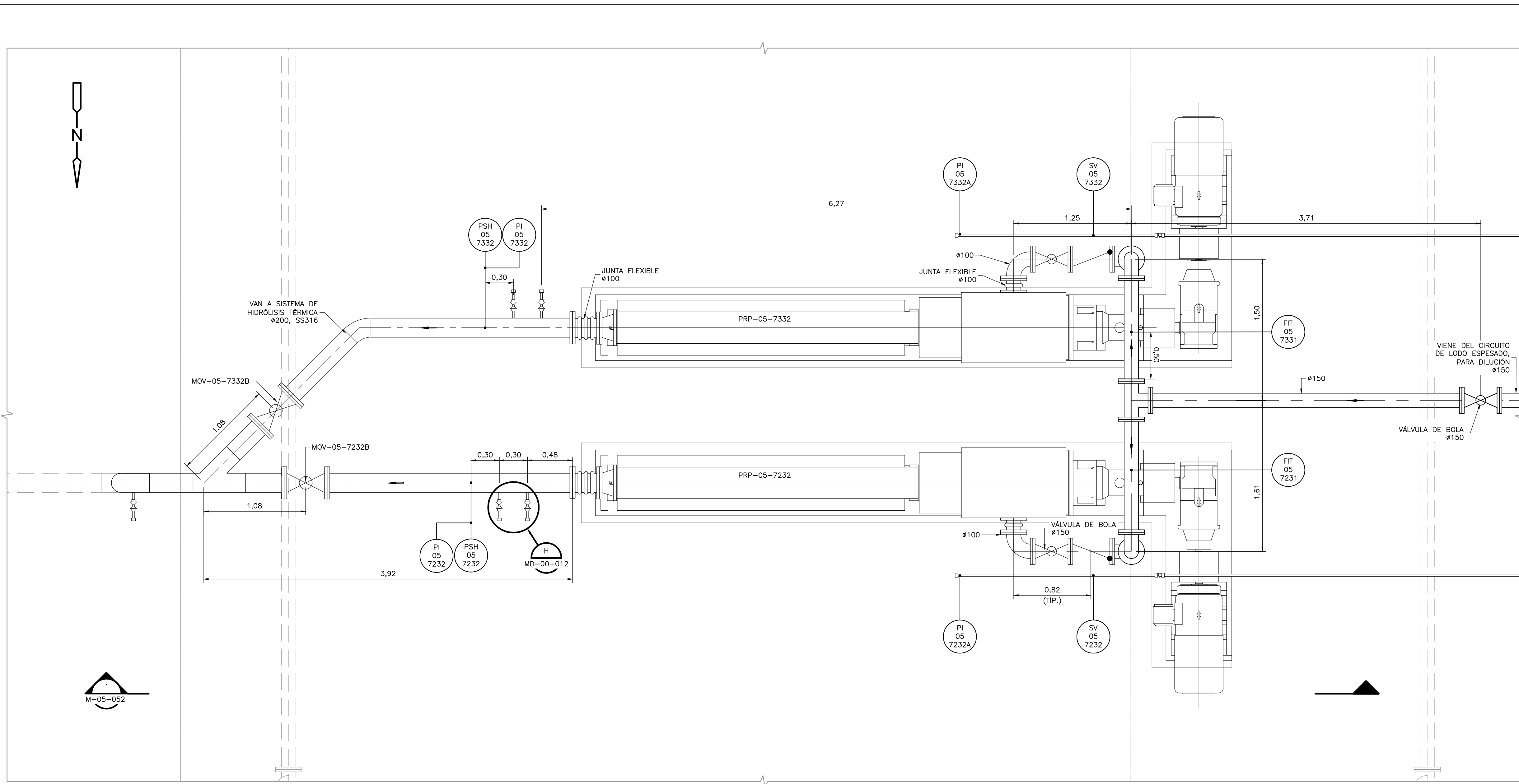
BOMBA DE LODOS PRE-DESHDRATADOS DETALLE C 1=25 M-05-041
