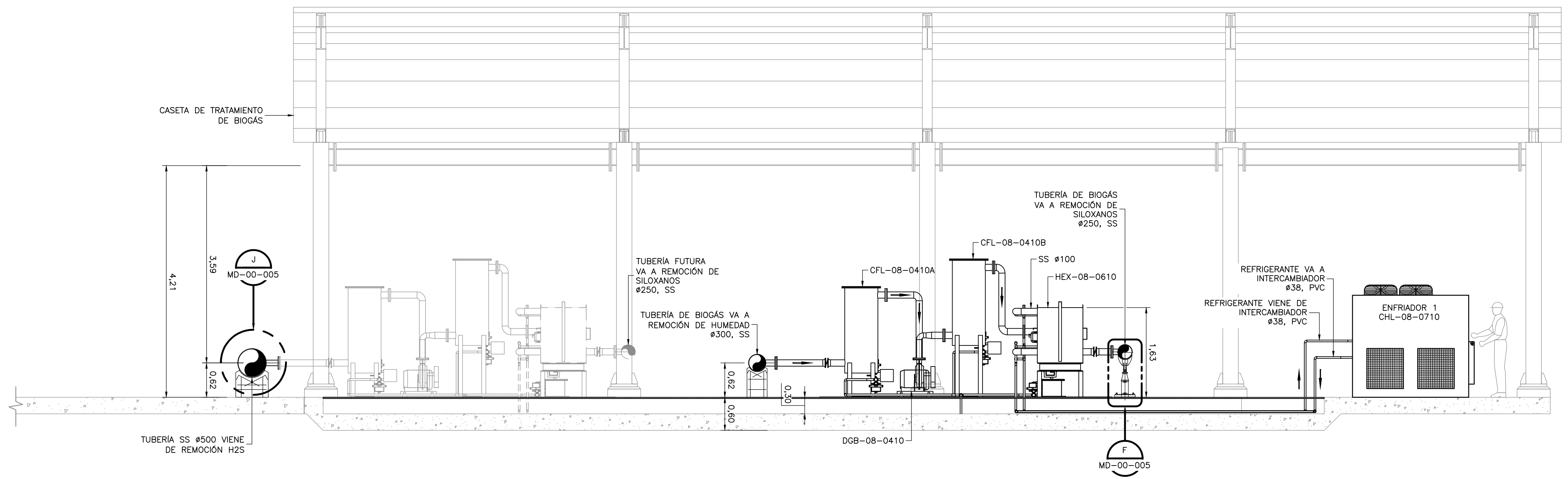
SECCIÓN 2 1=50 M-08-002
