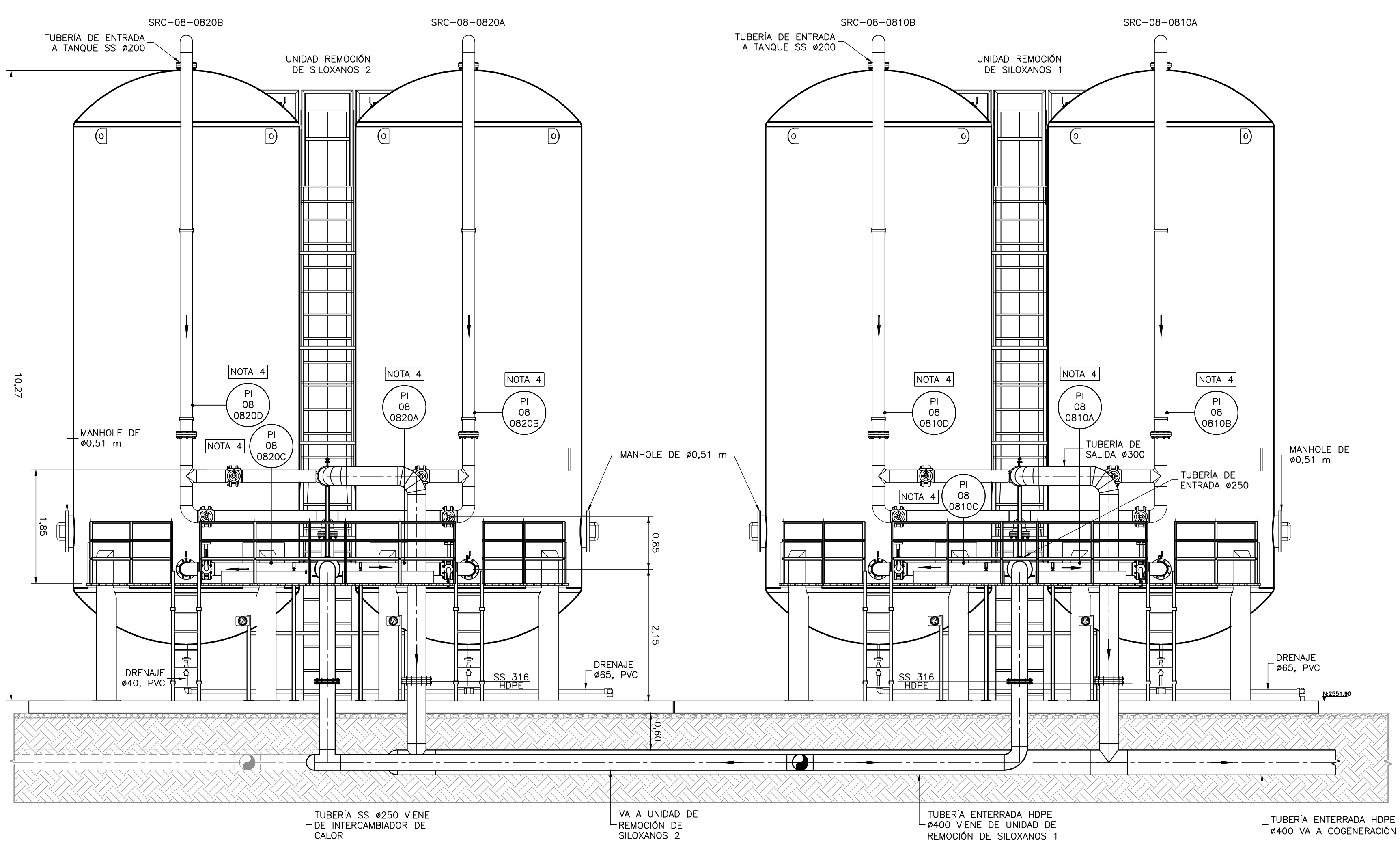
SECCIÓN 1 1=50 M-08-002
