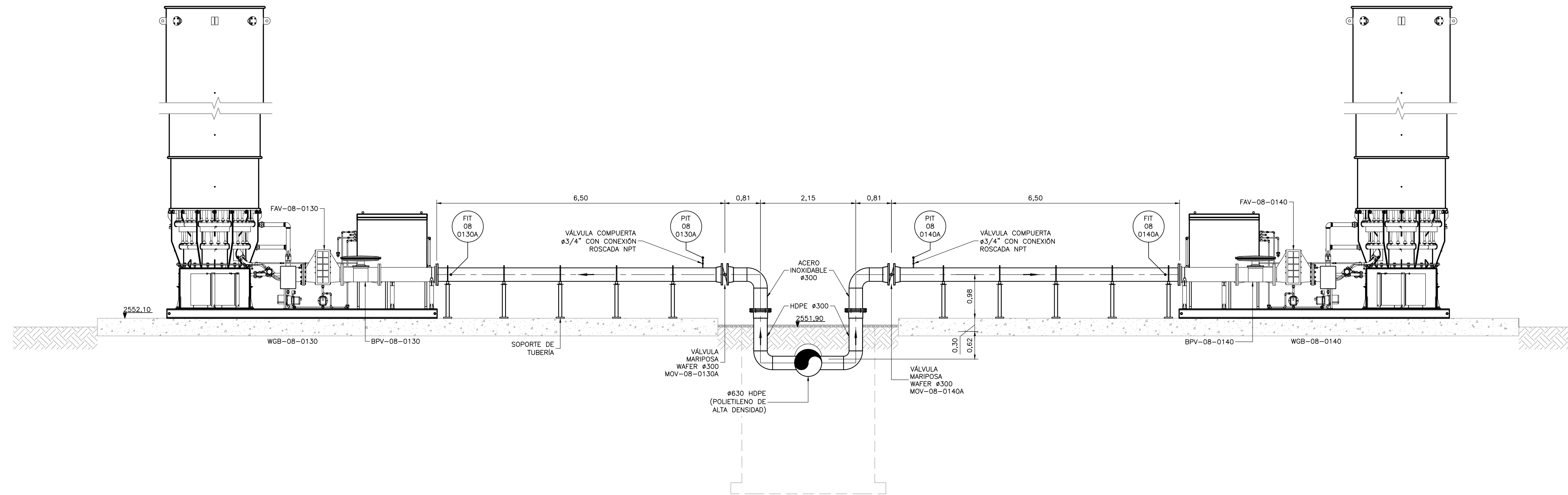
SECCIÓN 1 1=50 M-08-023
