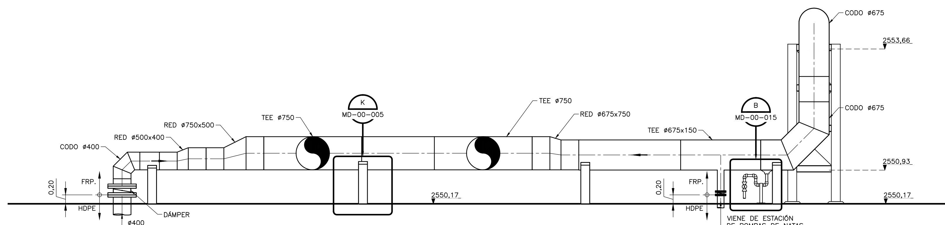
SECCIÓN 1 1=50 M-10-061
