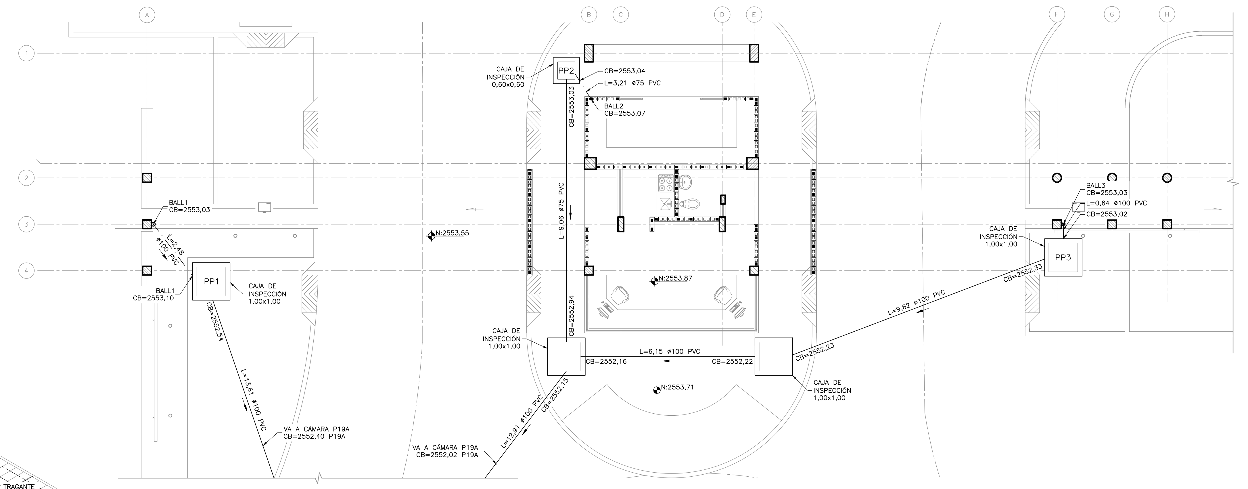
PLANTA CUBIERTA PORTERIA ADMINISTRACIÓN
