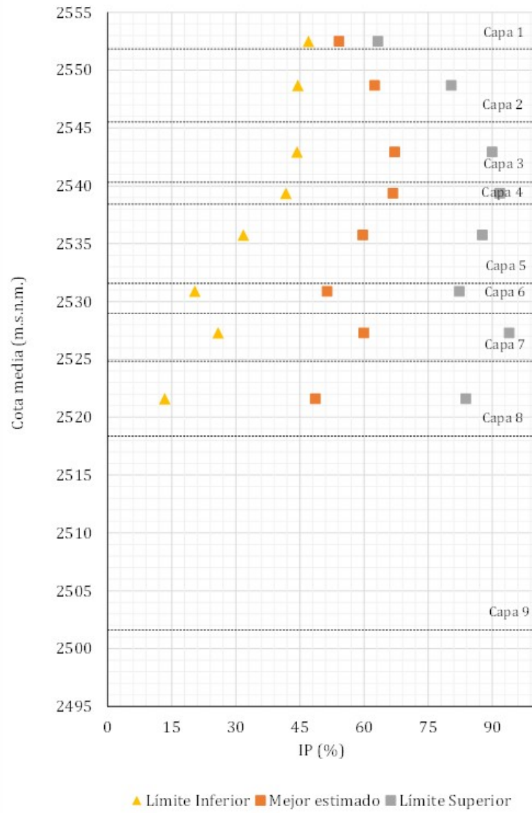
Valores de IP para los estratos de suelo de la PTAR Canoas
