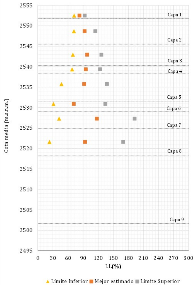
Valores de LL para los estratos de suelo de la PTAR Canoas
