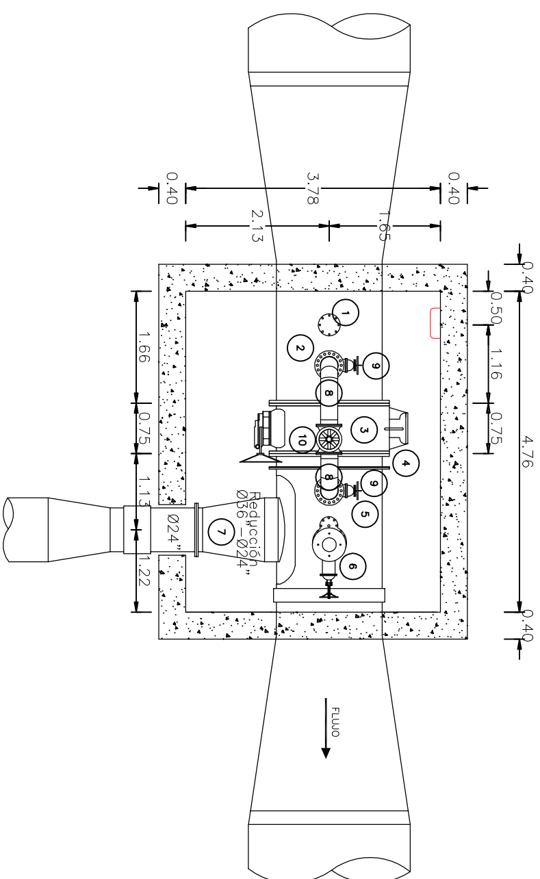
PLANTA CÁMARA VÁLVULA V-39
