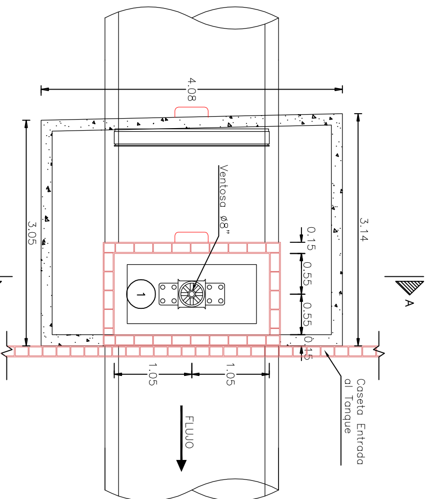
PLANTA CÁMARA VENTOSA
