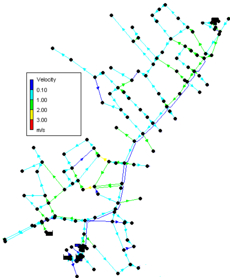
DEMANDA MAXIMA
