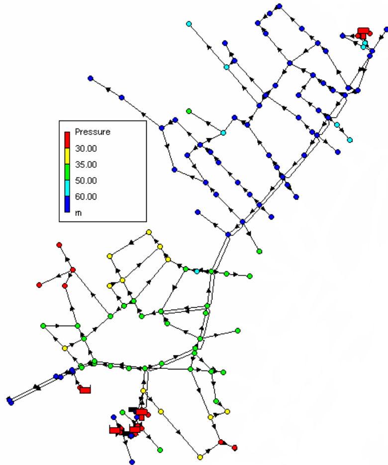
DEMANDA MAXIMA
