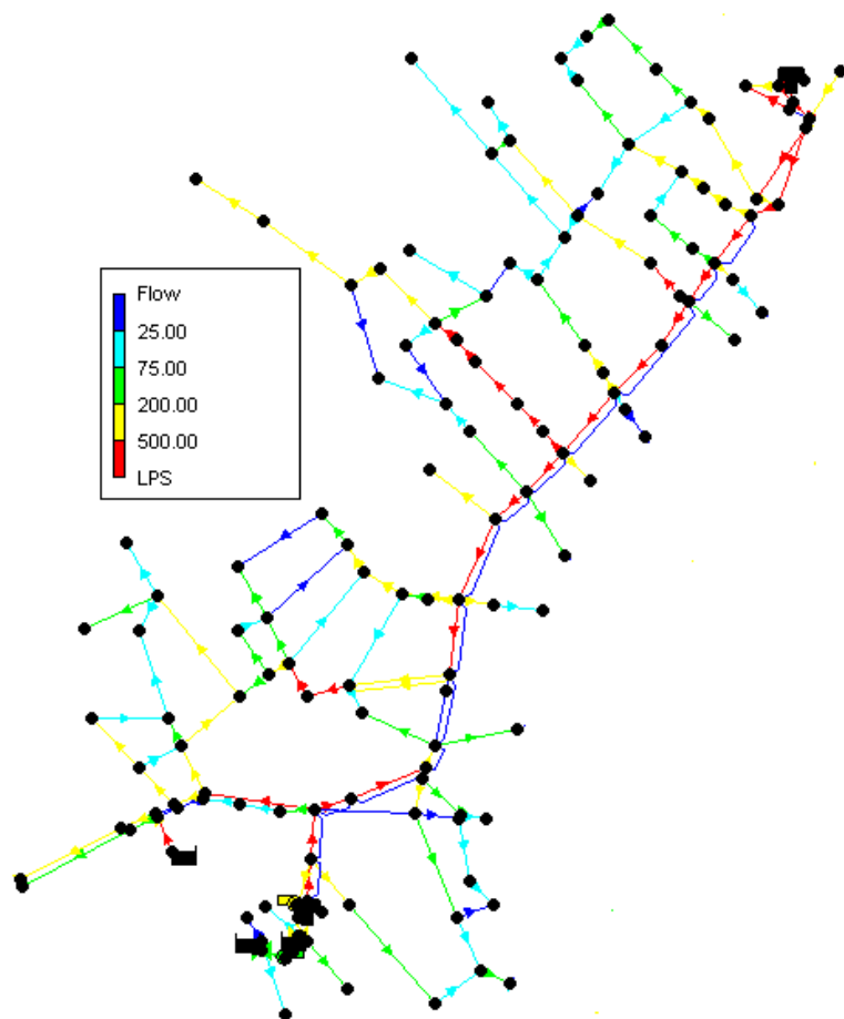
DEMANDA MAXIMA
