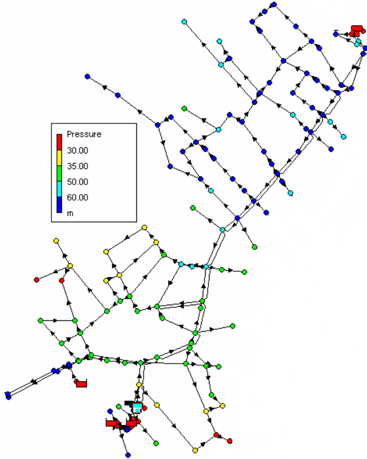
DEMANDA MAXIMA
