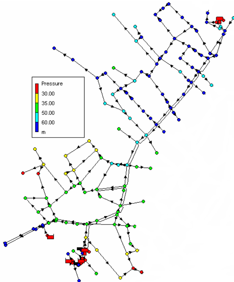
DEMANDA MAXIMA
