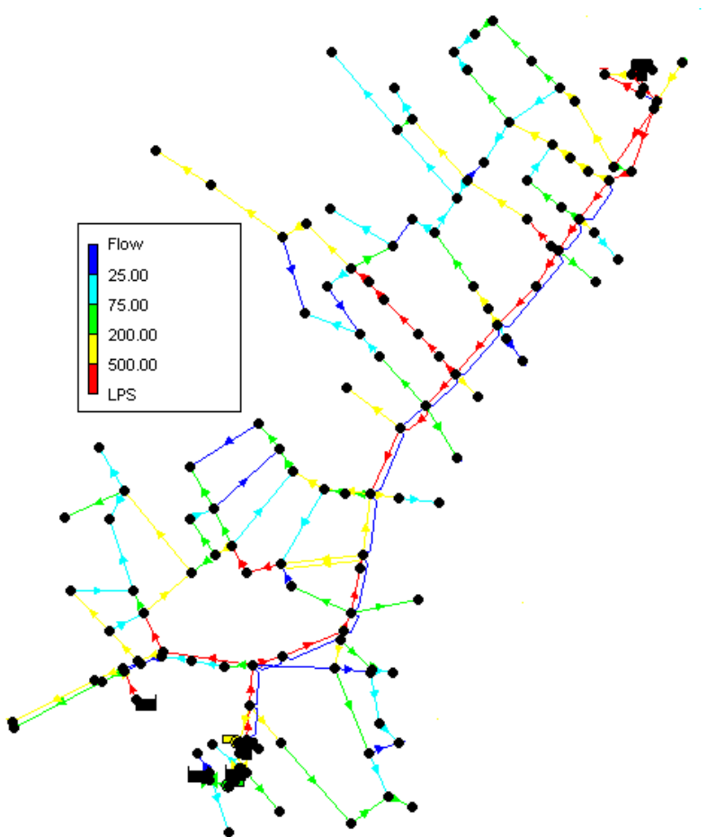
DEMANDA MAXIMA
