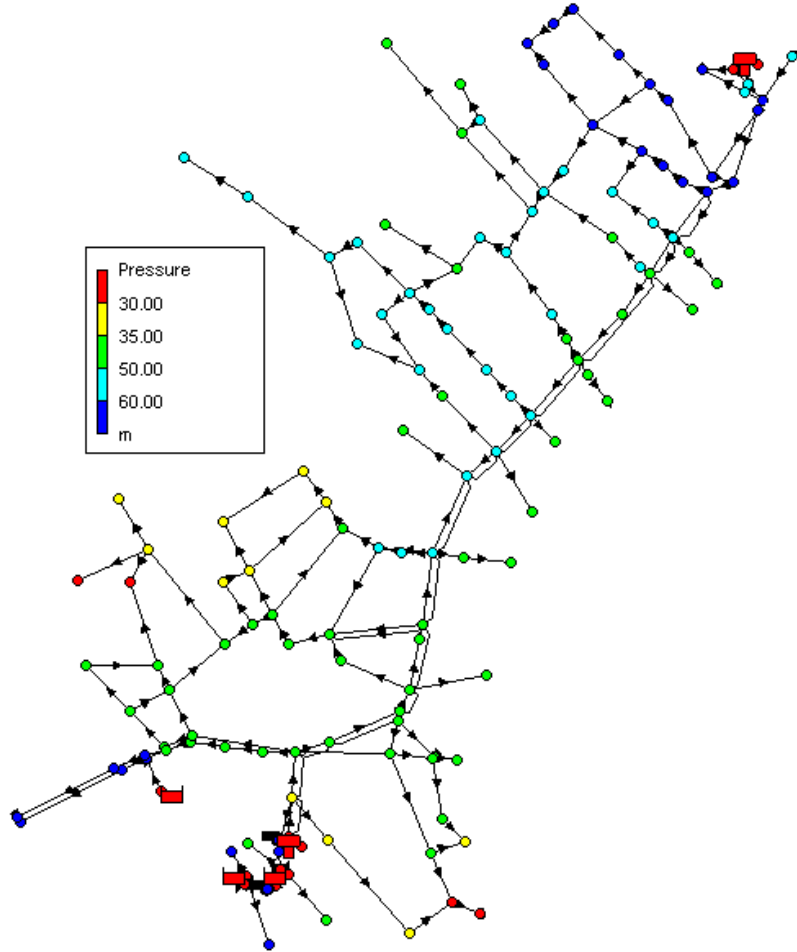
DEMANDA MAXIMA
