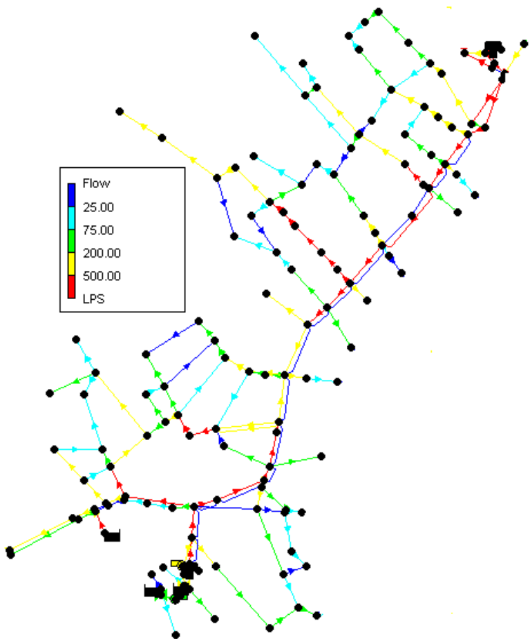
DEMANDA MAXIMA
