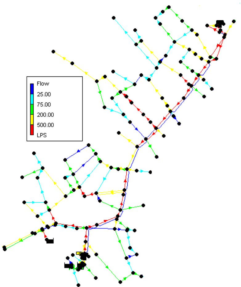
DEMANDA MAXIMA
