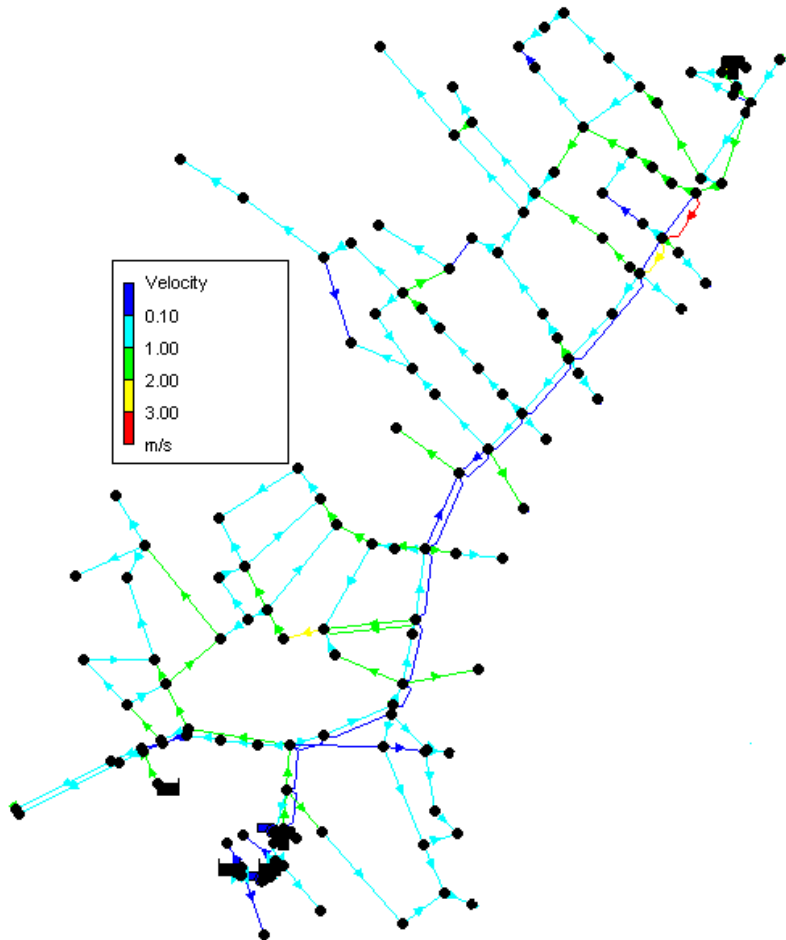
DEMANDA MAXIMA
