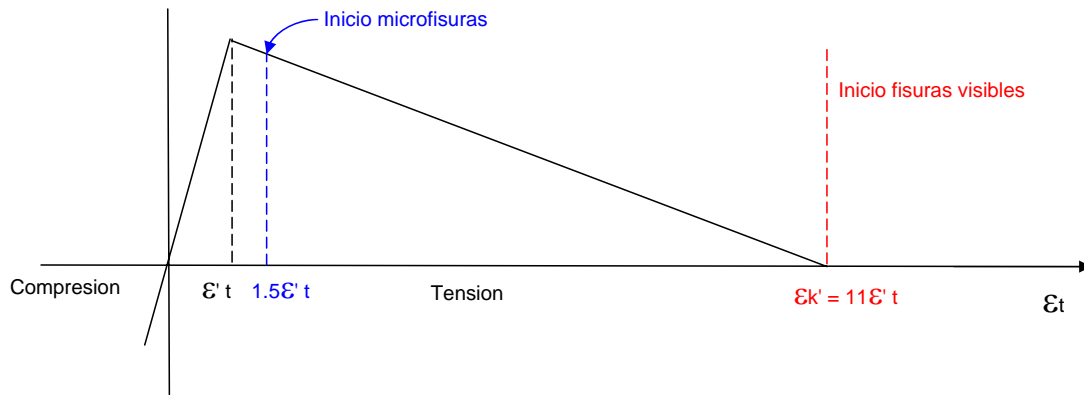
RELACION ESFUERZO-DEFORMACION PARA EL NUCLEO DE CONCRETO
