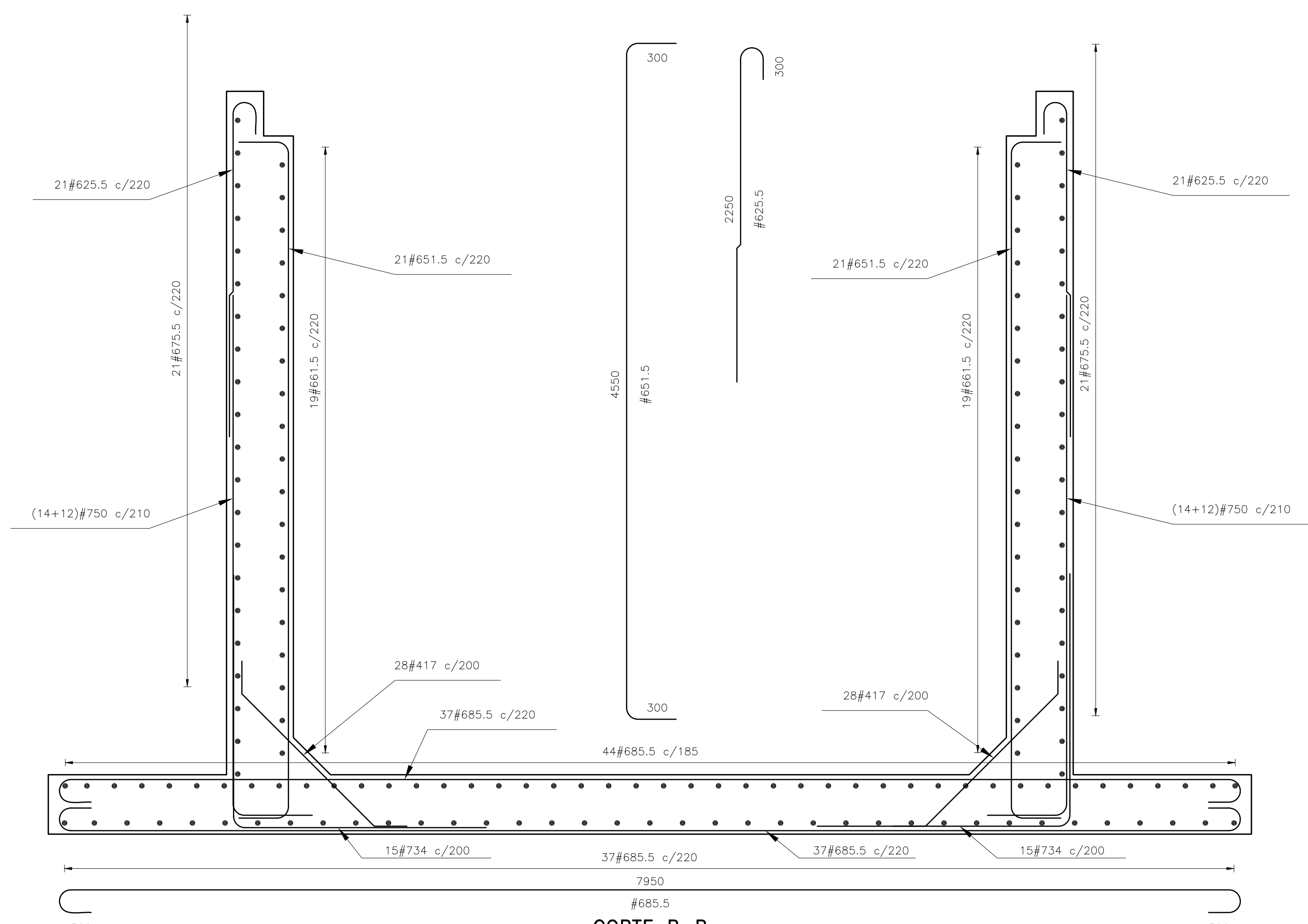
CORTE B-B REFUERZO MUROS LATERALES Y LOSA DE FONDO ESCALA 1:25
