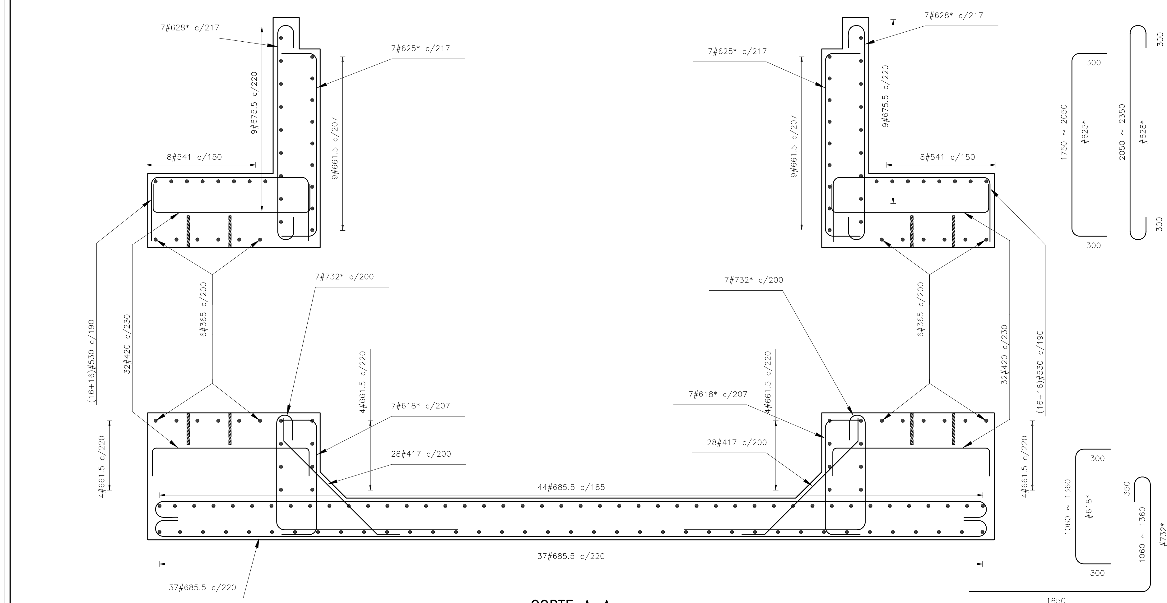
CORTE A-A REFUERZO MUROS, MUERTOS DE ANCLAJE Y LOSA DE FONDO ESCALA 1:25
